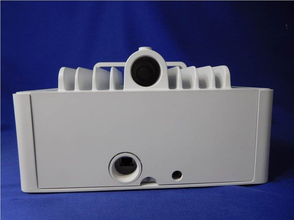
(163)EUT Photo
