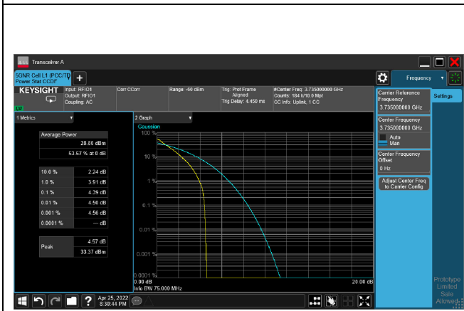
5G NR n77_CH649000_70M_1RB_pi/2 BPSK_Ratio
