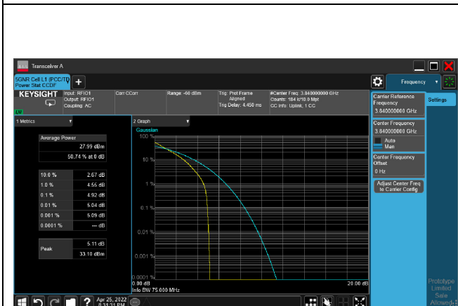
5G NR n77_CH656000_70M_1RB_QPSK_Ratio
