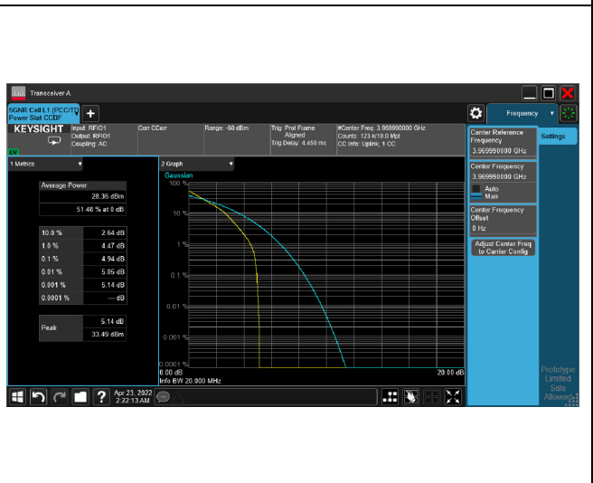
5G NR n77_CH664666_20M_1RB_QPSK_Ratio
