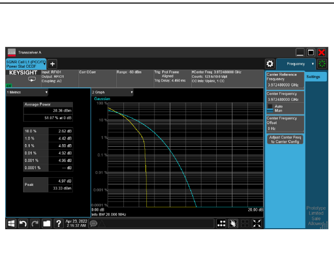
5G NR n77_CH664832_15M_1RB_QPSK_Ratio
