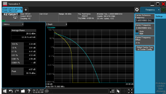
5G NR n77_CH632334_70M_1RB_16-QAM_Ratio
