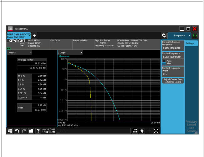
5G NR n77_CH633334 _100M_1RB_QPSK_Ratio
