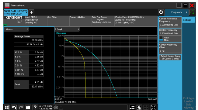
5G NR n77_CH633334_70M_1RB_16-QAM_Ratio
