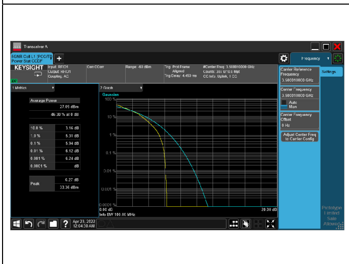
5G NR n77_CH633334 _100M_1RB_16-QAM_Ratio
