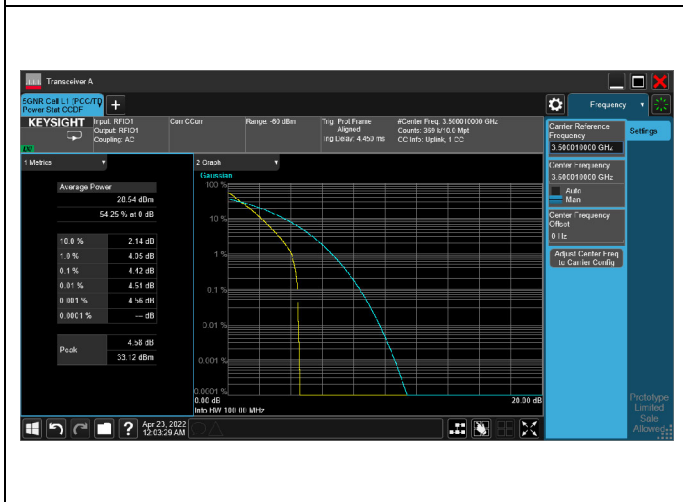
5G NR n77_CH633334 _100M_1RB_16-QAM_Ratio
