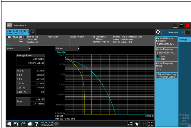
5G NR n77_CH632000_60M_1RB_pi/2 BPSK_Ratio
