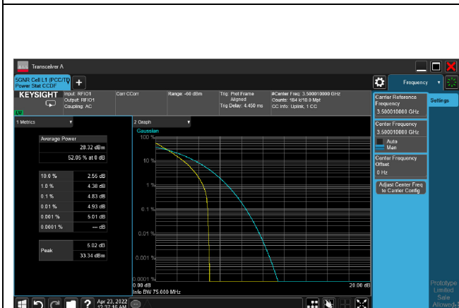
5G NR n77_CH633334_60M_1RB_QPSK_Ratio
