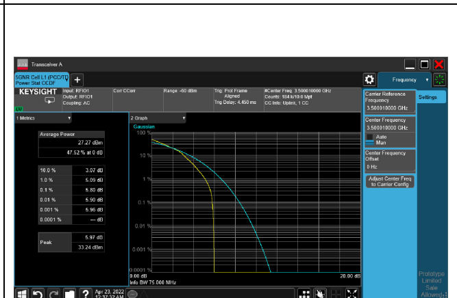
5G NR n77_CH633334_60M_1RB_16-QAM_Ratio
