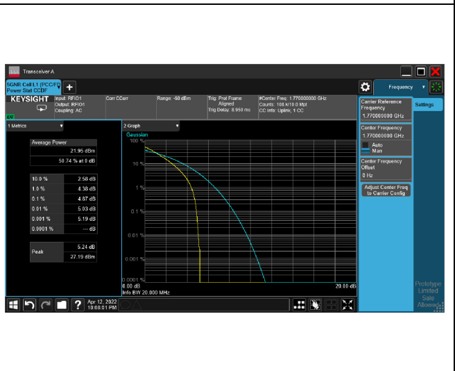
5G NR n66_CH354000_20M_1RB_QPSK_Ratio
