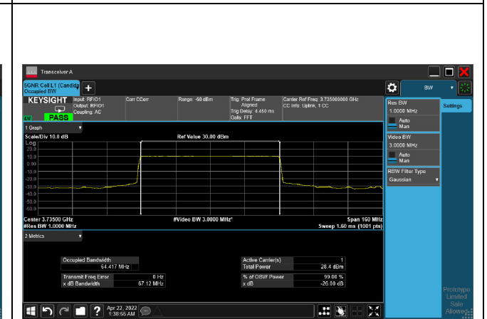
QPSK_CH649000_70M
