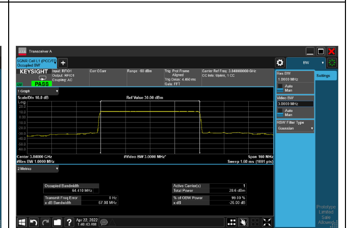
pi/2-BPSK_CH656000_70M
