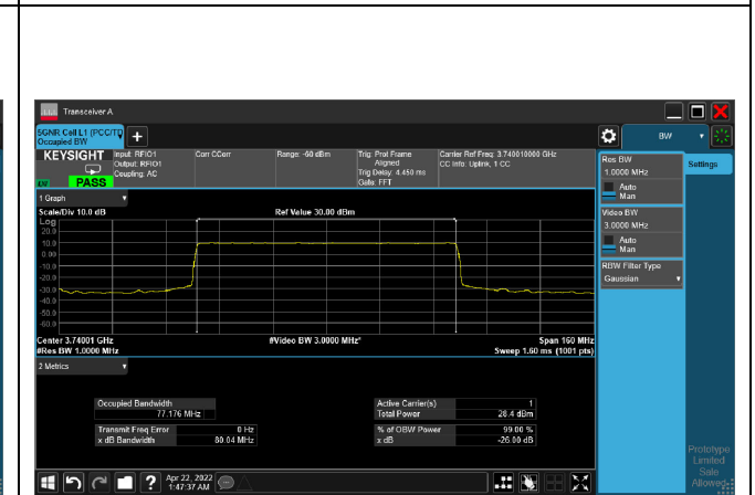
QPSK_CH649334_80M
