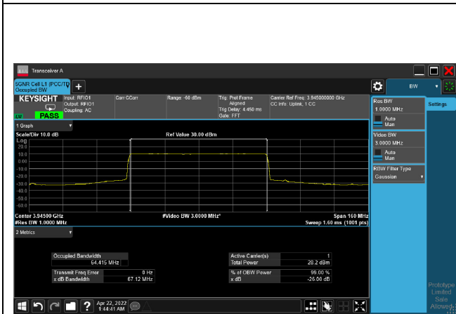
pi/2-BPSK_CH663000_70M
