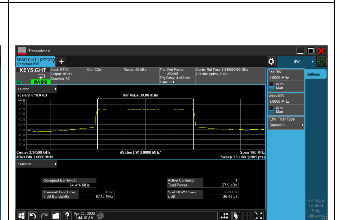
QPSK_CH663000_70M
