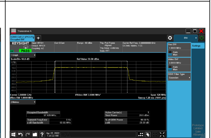
pi/2-BPSK_CH656000_60M
