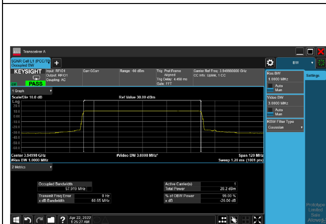
pi/2-BPSK_CH663332_60M
