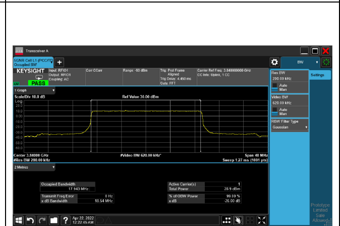
pi/2-BPSK_CH656000_20M
