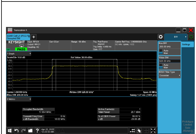
pi/2-BPSK_CH664666_20M
