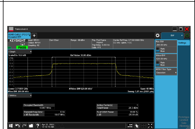
QPSK_CH647334_20M
