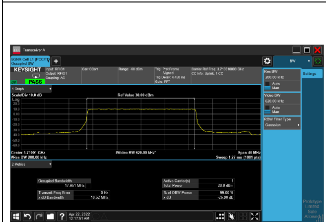
pi/2-BPSK_CH647334_20M
