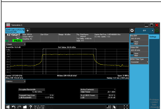
pi/2-BPSK_CH664832_15M
