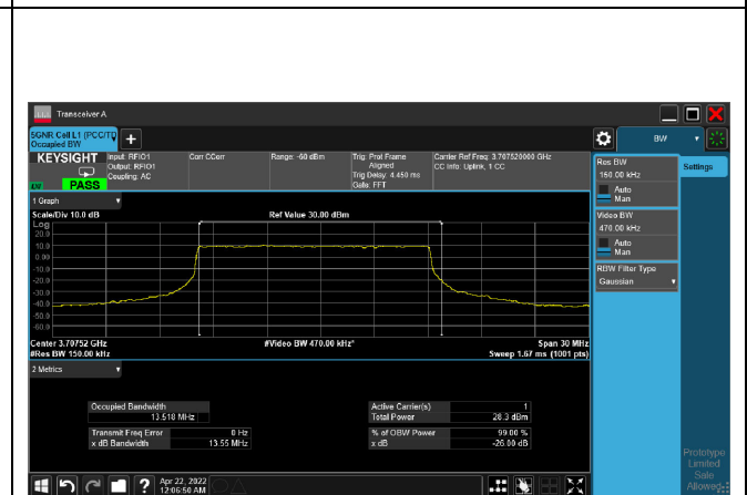
QPSK_CH647168_15M
