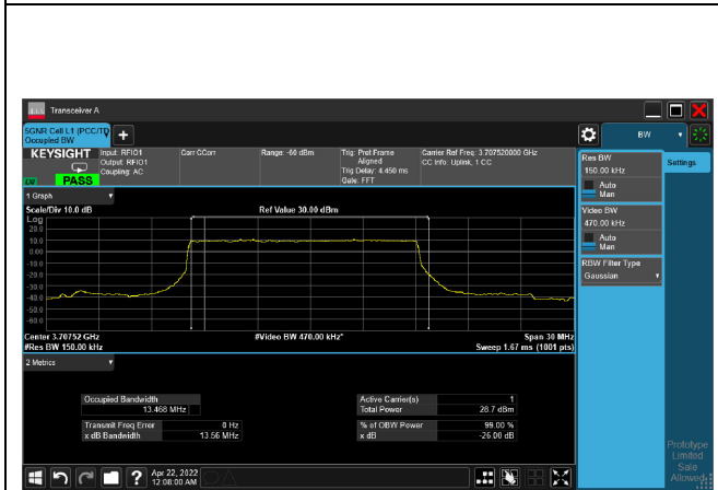
pi/2-BPSK_CH647168_15M
