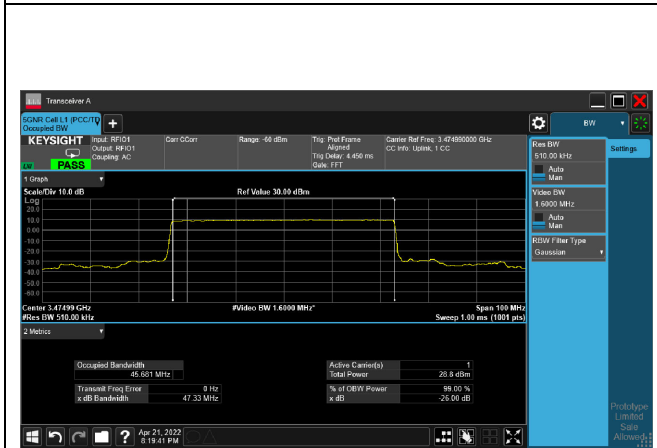
pi/2-BPSK_CH631666_50M
