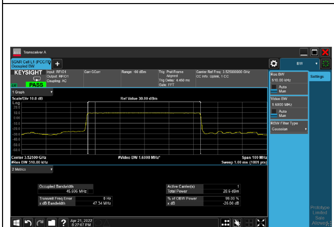
pi/2-BPSK_CH635000_50M
