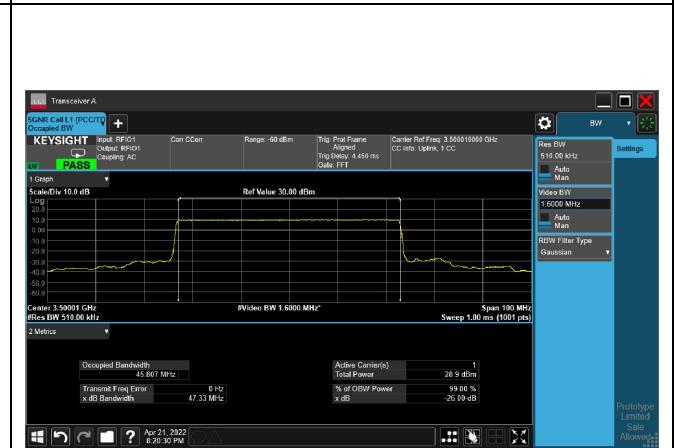
pi/2-BPSK_CH633334_50M
