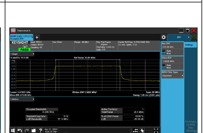
QPSK_CH631334_40M
