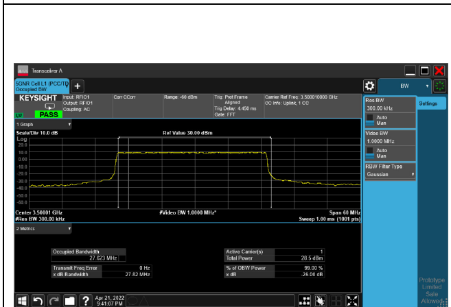
QPSK_CH63333430M
