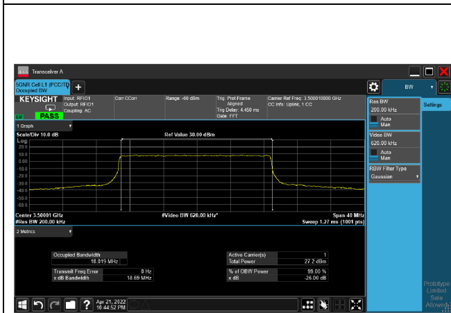
64QAM_CH633334_20M
