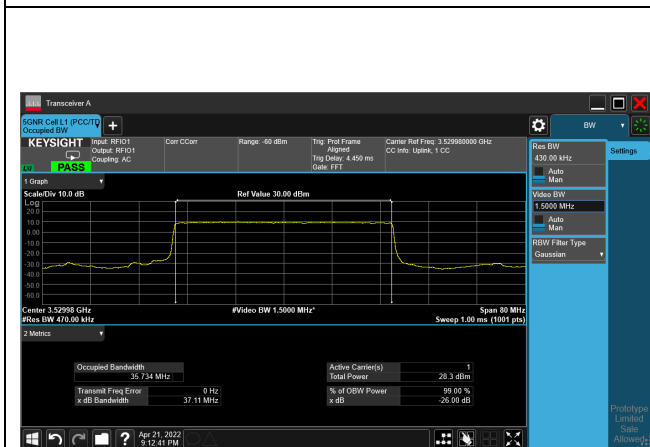
pi/2-BPSK_CH635332_40M
