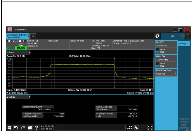
pi/2-BPSK_CH631000_30M
