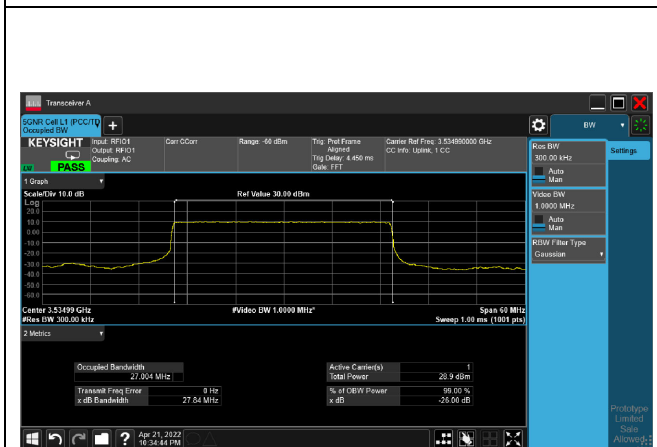
pi/2-BPSK_CH635666_30M
