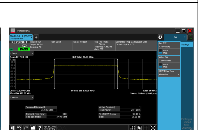
QPSK_CH635332_40M
