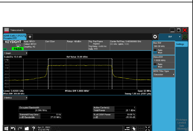
QPSK_CH631000_30M
