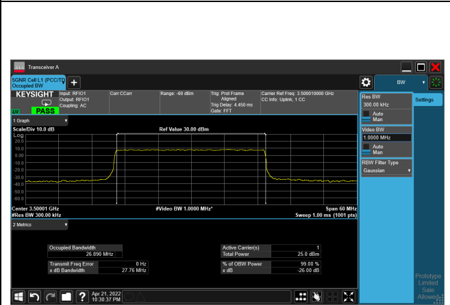
256QAM_CH633334_30M
