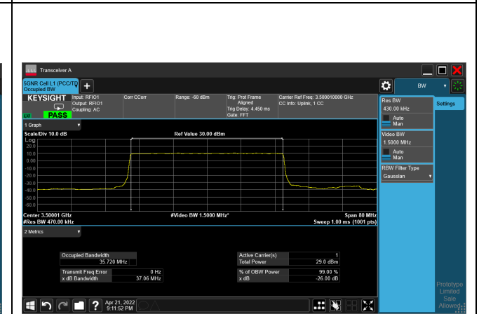
pi/2-BPSK_CH633334_40M
