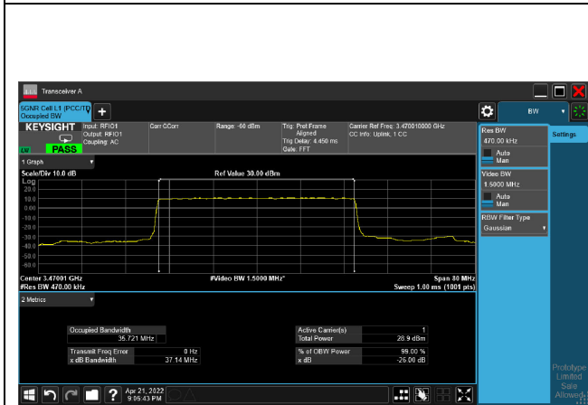
pi/2-BPSK_CH631334_40M
