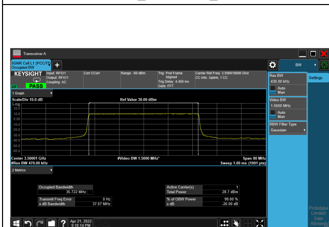
QPSK_CH633334_40M
