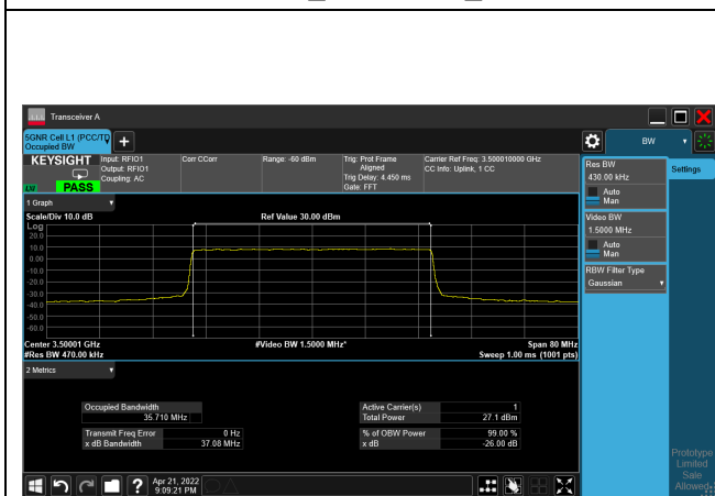
64QAM_CH633334_40M
