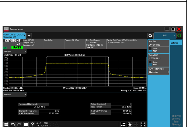
QPSK_CH635666_30M
