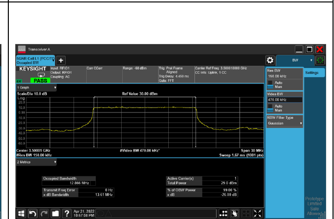
pi/2-BPSK_CH 633334_15M
