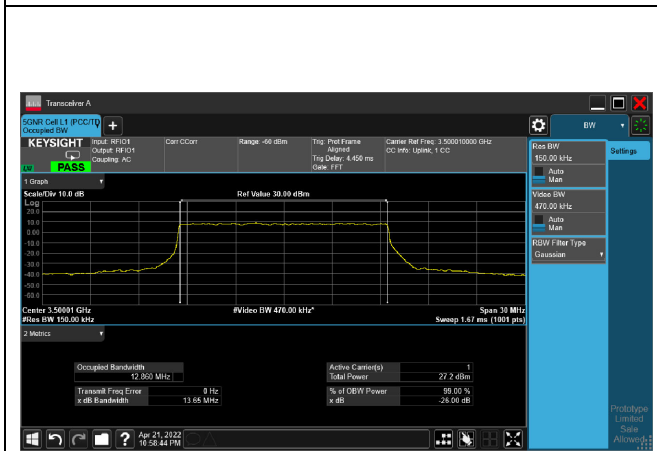
64QAM_CH633334_15M
