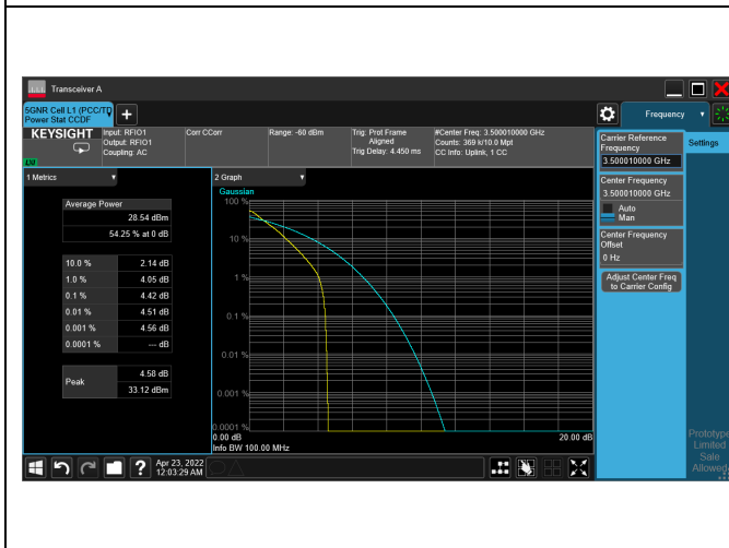
5G NR n77_CH633334 _100M_1RB_16-QAM_Ratio
