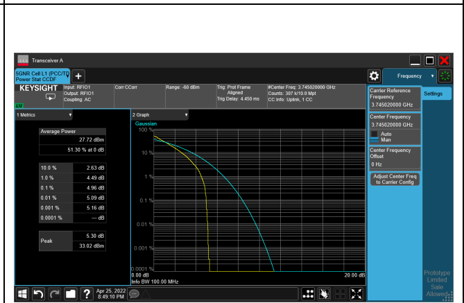
5G NR n77_CH649668_90M_1RB_QPSK_Ratio
