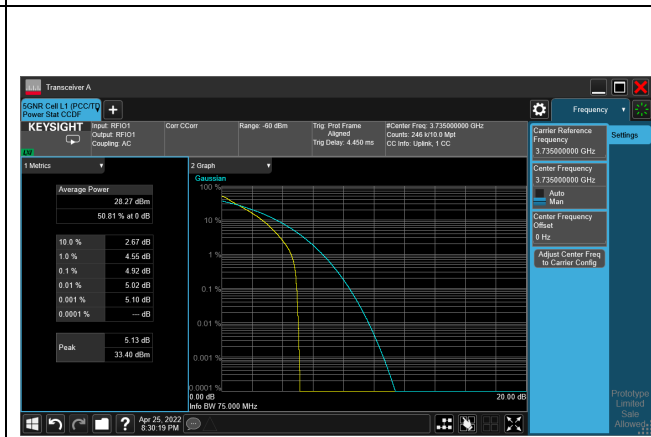
5G NR n77_CH649000_70M_1RB_QPSK_Ratio
