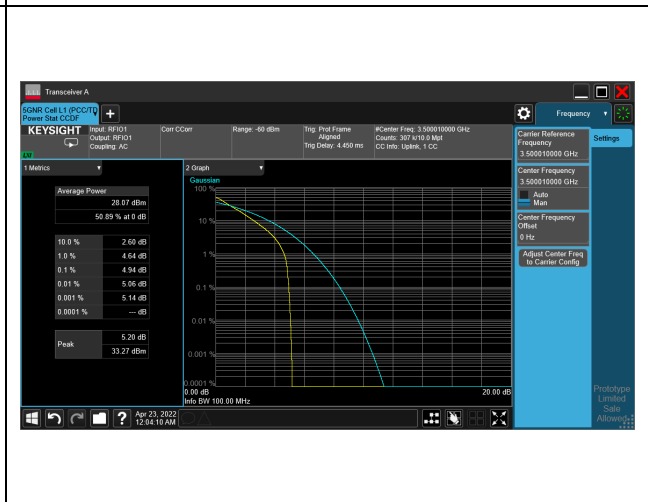
5G NR n77_CH633334 _100M_1RB_QPSK_Ratio
