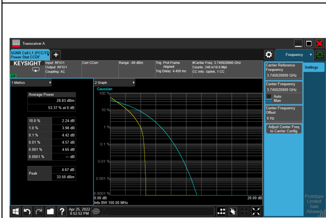
5G NR n77_CH649668_90M_1RB_pi/2 BPSK_Ratio
