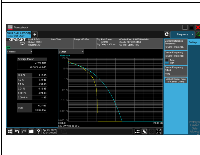
5G NR n77_CH633334 _100M_1RB_16-QAM_Ratio
