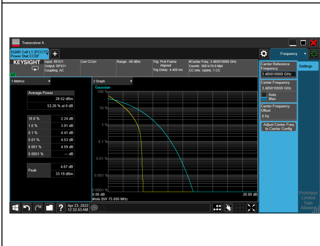
5G NR n77_CH632334_70M_1RB_16-QAM_Ratio
