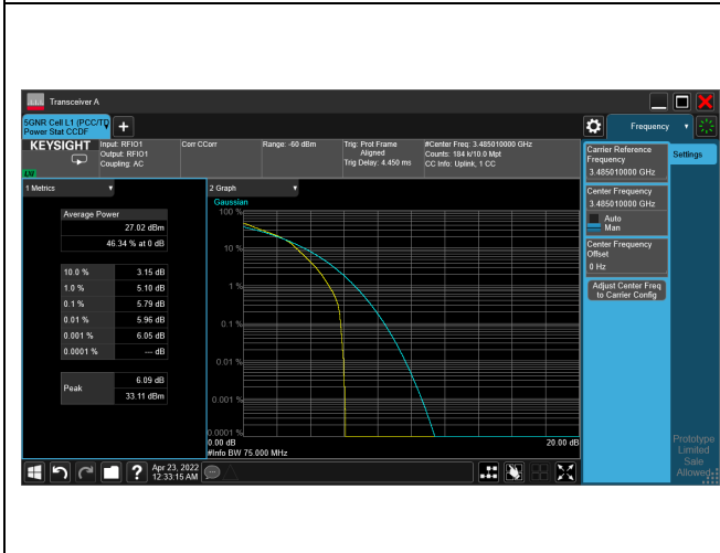
5G NR n77_CH633334_70M_1RB_QPSK_Ratio
