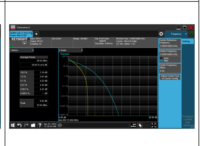
5G NR n77_CH633334_60M_1RB_16-QAM_Ratio
