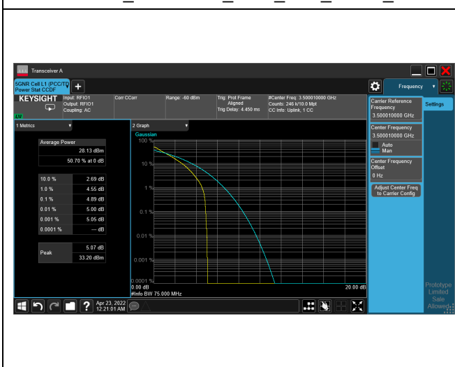
5G NR n77_CH633334_70M_1RB_QPSK_Ratio
