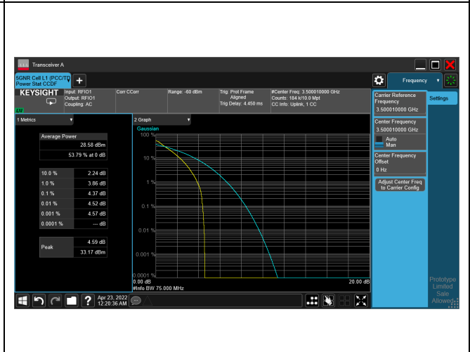
5G NR n77_CH633334_70M_1RB_16-QAM_Ratio
