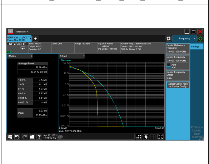
5G NR n77_CH633334_70M_1RB_16-QAM_Ratio
