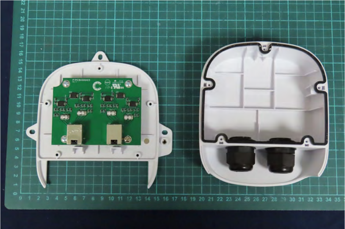
(72) EUT Photo
