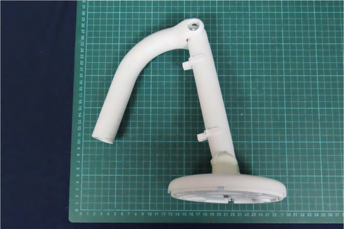
(77) EUT Photo
