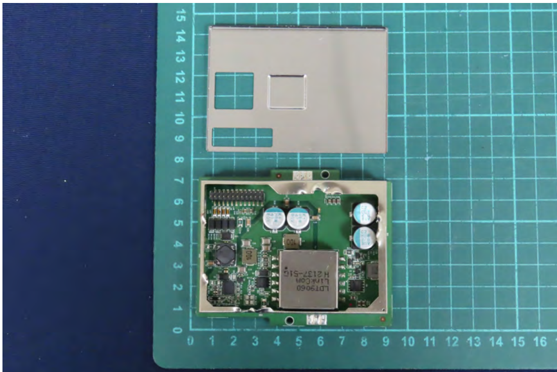
(44) EUT Photo
