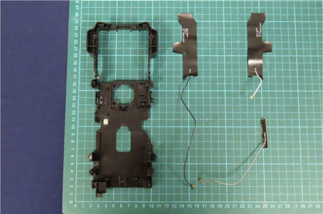
(50) EUT Photo
