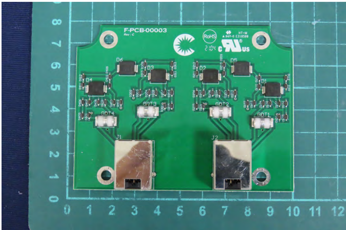
(75) EUT Photo
