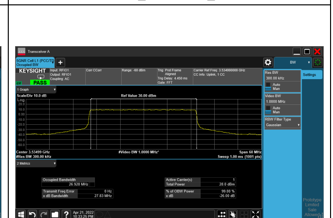
QPSK_CH635666_30M
