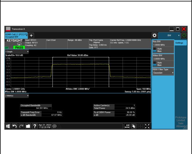
256QAM_CH633334_70M
