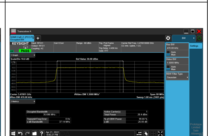
QPSK_CH631334_40M
