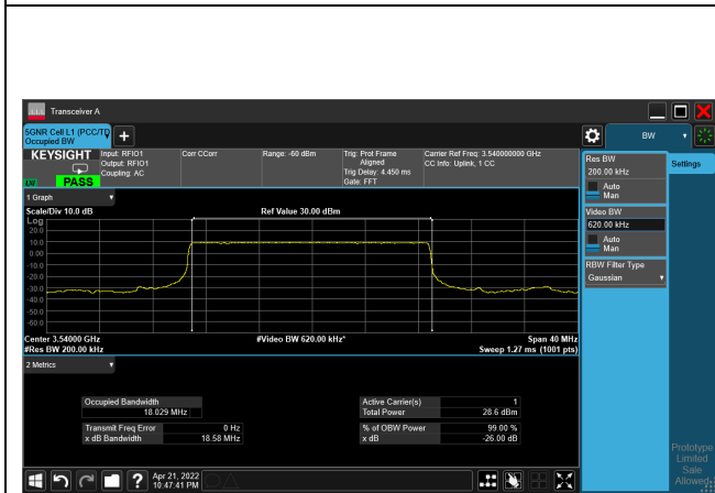
pi/2-BPSK_CH636000_20M
