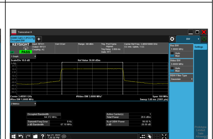
QPSK_CH632334_70M
