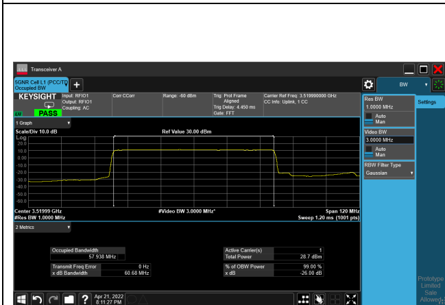
pi/2-BPSK_CH634666_60M
