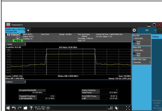
pi/2-BPSK_CH632334_70M
