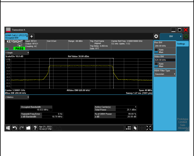
256QAM_CH633334_20M
