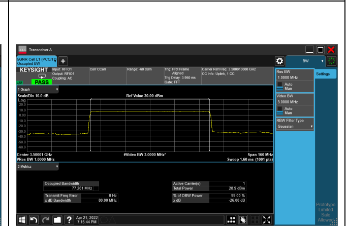
pi/2-BPSK_CH633334_80M
