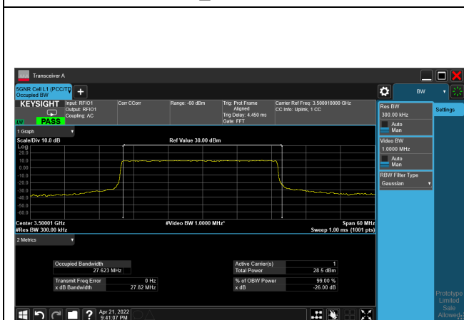
QPSK_CH63333430M
