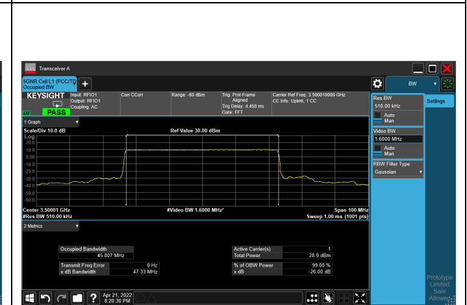
pi/2-BPSK_CH633334_50M
