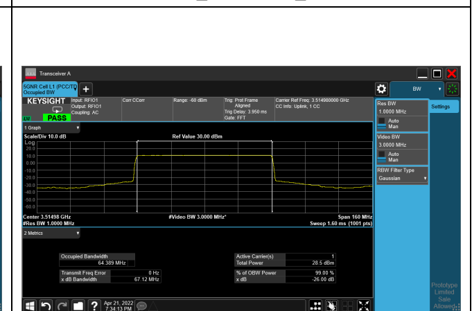
QPSK_CH634332_70M
