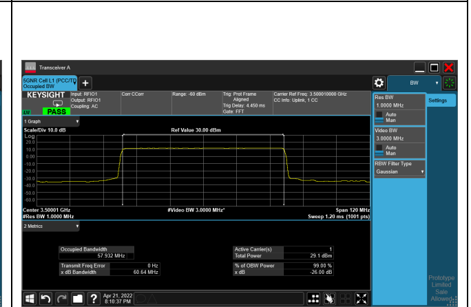
pi/2-BPSK_CH633334_60M
