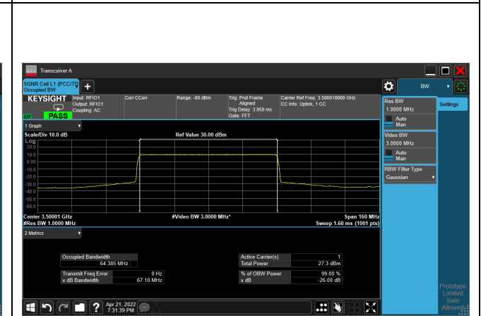
16QAM_CH633334_70M
