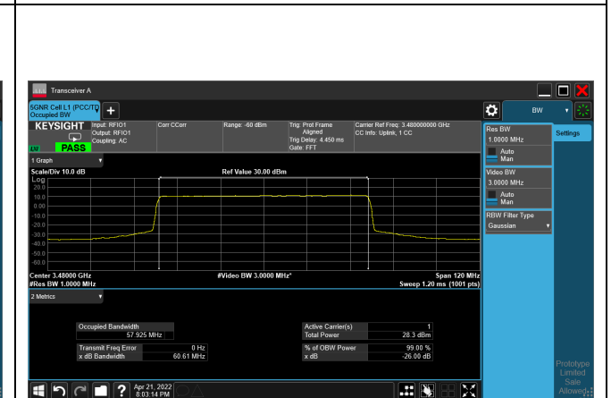
QPSK_CH632000_60M
