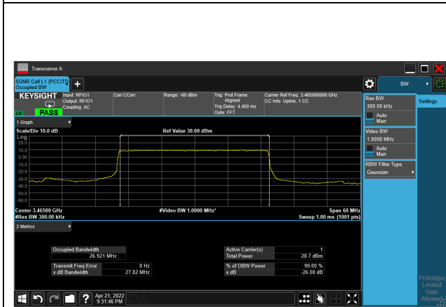
pi/2-BPSK_CH631000_30M
