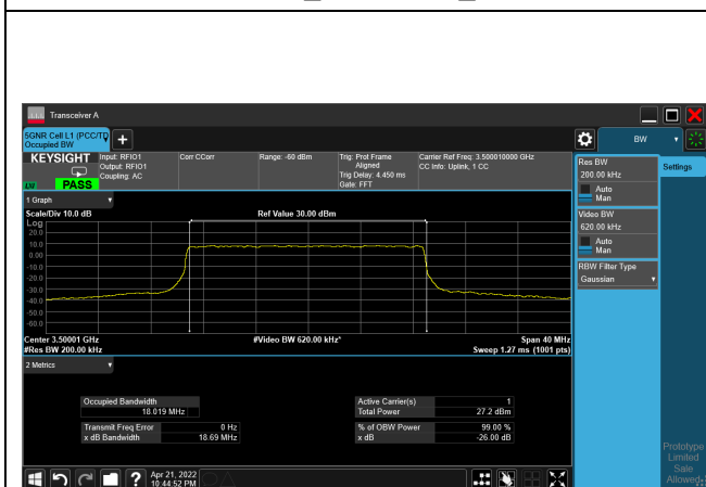
64QAM_CH633334_20M
