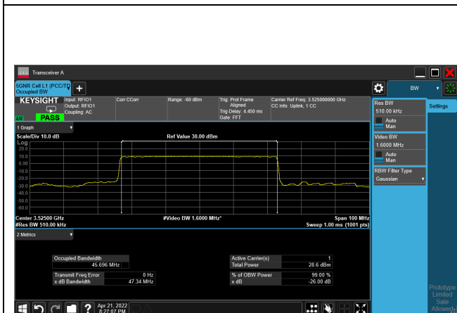
pi/2-BPSK_CH635000_50M
