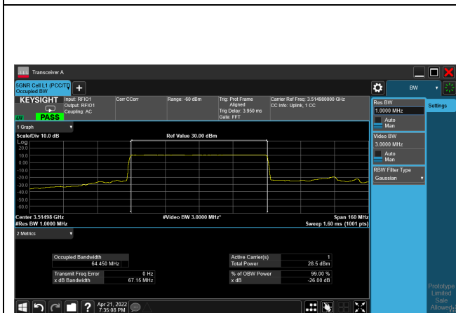
pi/2-BPSK_CH634332_70M
