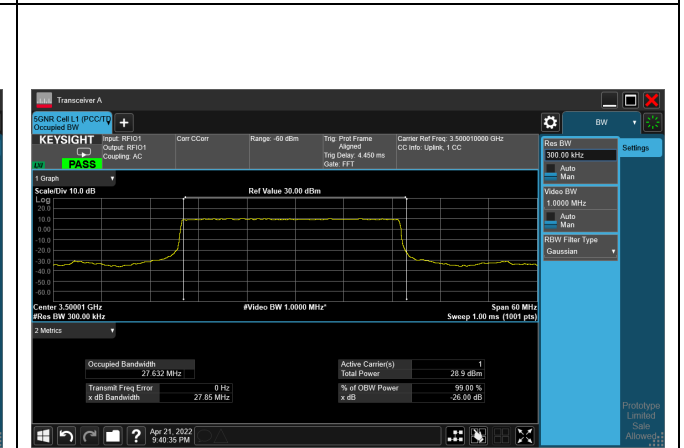
pi/2-BPSK_CH633334_30M
