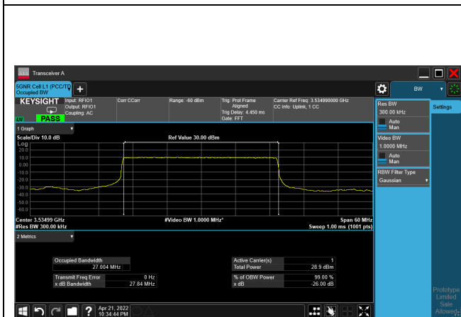
pi/2-BPSK_CH635666_30M
