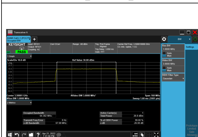
64QAM_CH633334_70M
