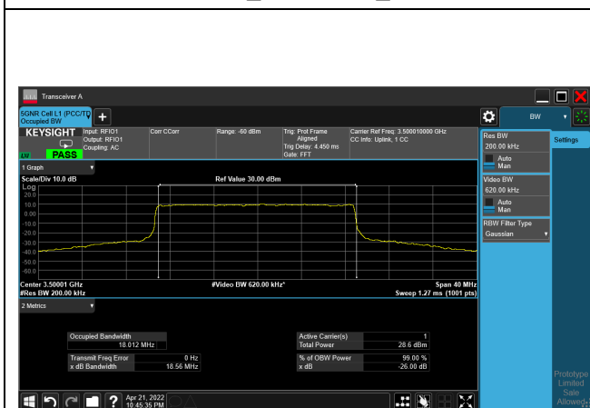
QPSK_CH633334_20M
