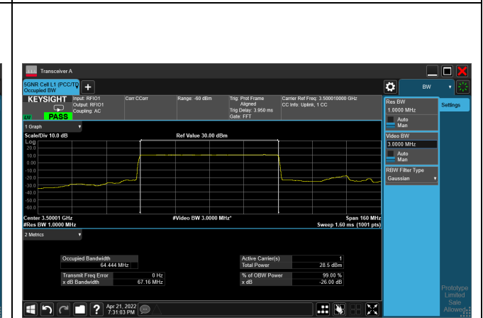
pi/2-BPSK_CH633334_70M
