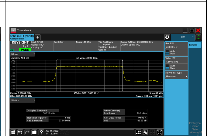
pi/2-BPSK_CH633334_40M
