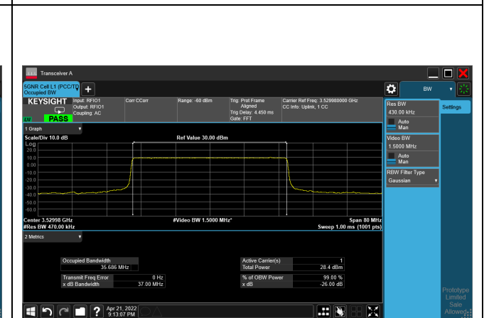
QPSK_CH635332_40M
