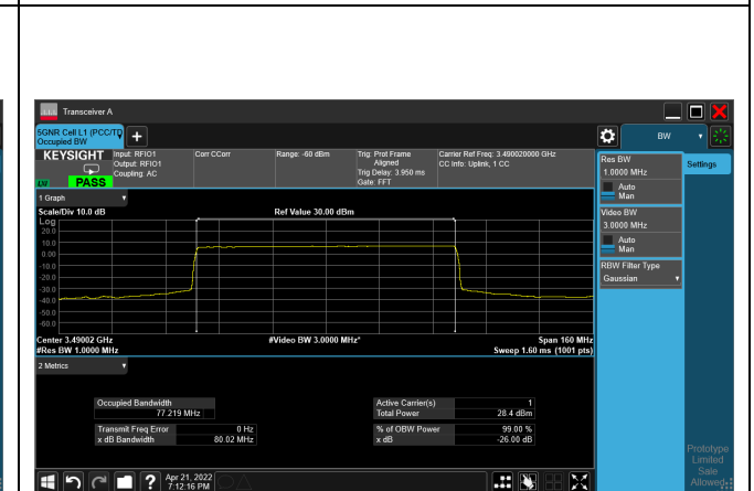
QPSK_CH632668_80M
