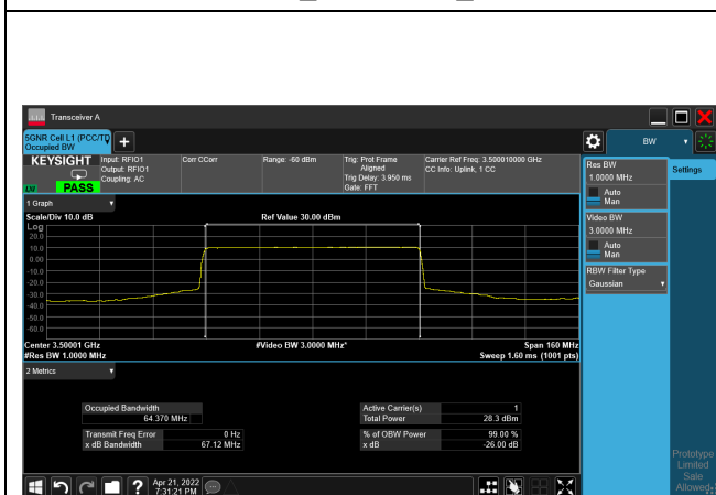
QPSK_CH633334_70M
