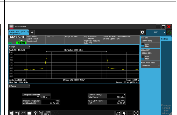
QPSK_CH634000_80M
