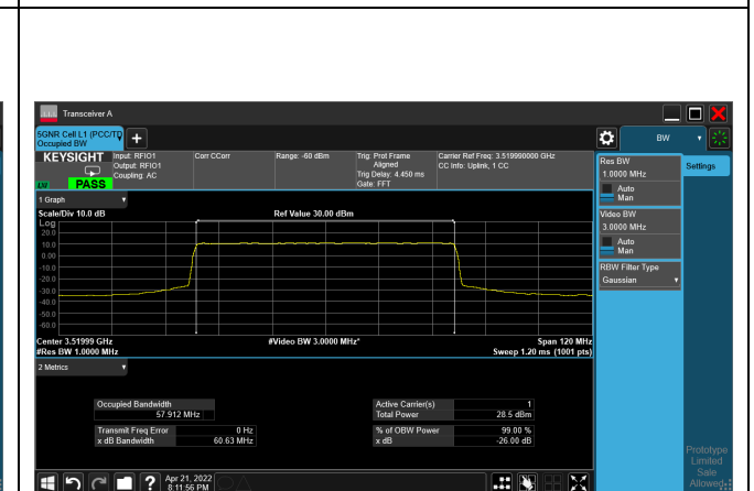
QPSK_CH634666_60M
