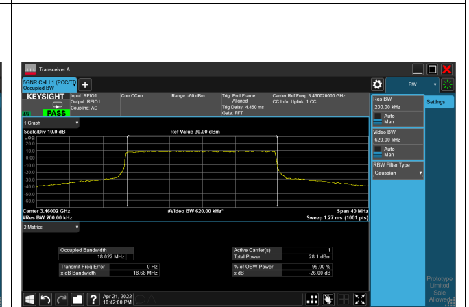
QPSK_CH630668_20M
