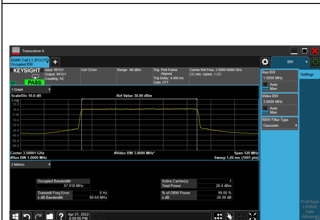
QPSK_CH633334_60M
