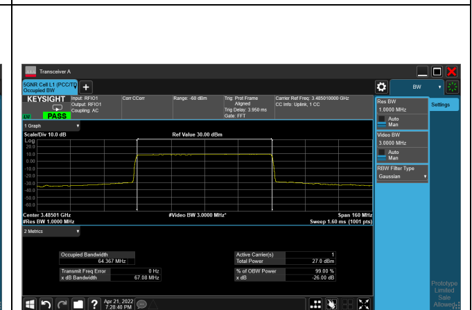
64QAM_CH632334_70M
