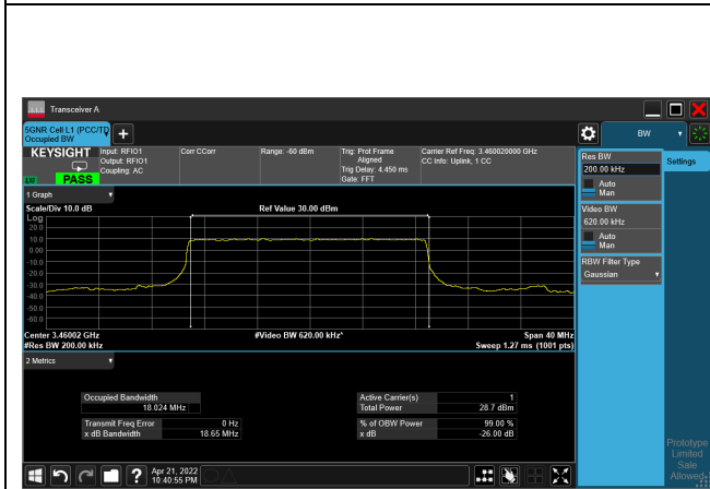
pi/2-BPSK_CH630668_20M
