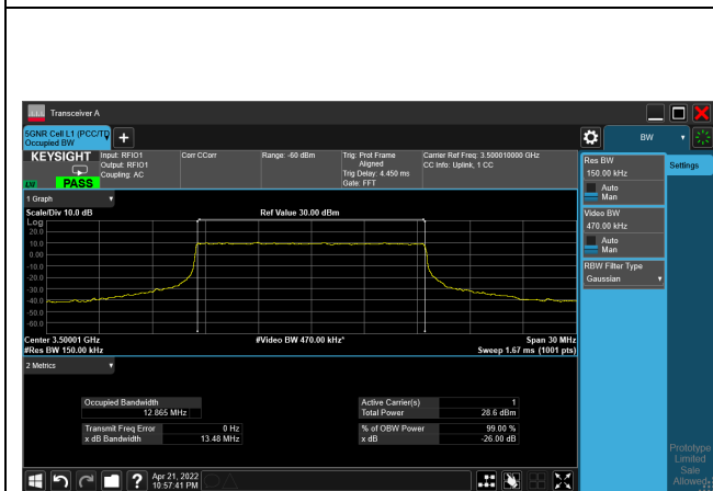
QPSK_CH 633334_15M
