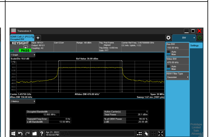
QPSK_CH630500_15M
