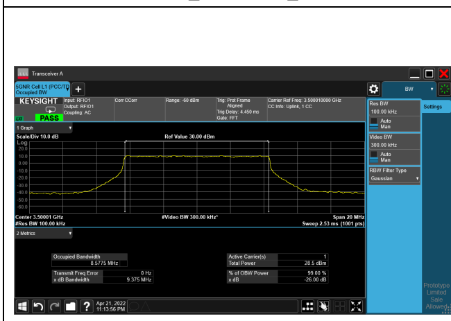
QPSK_CH633334_10M
