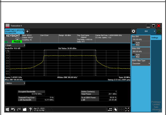
QPSK_CH630334_10M
