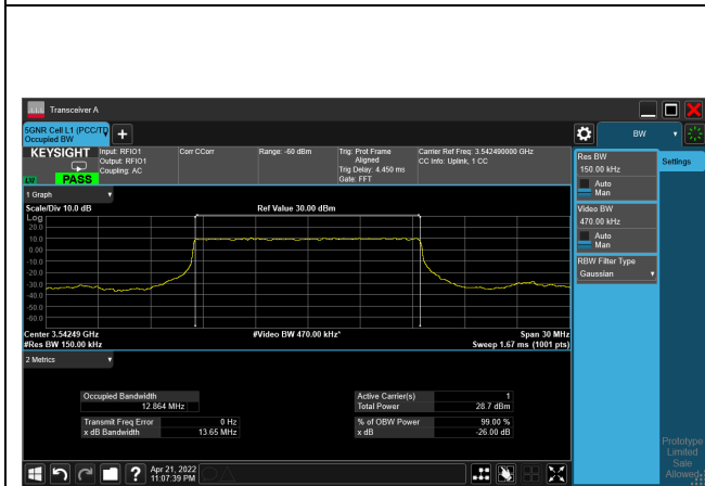
pi/2-BPSK_CH 636166_15M
