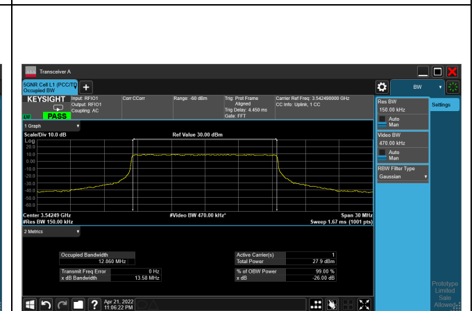
QPSK_CH 636166_15M
