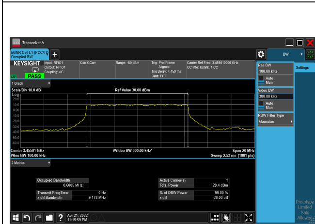
pi/2-BPSK_CH630334_10M
