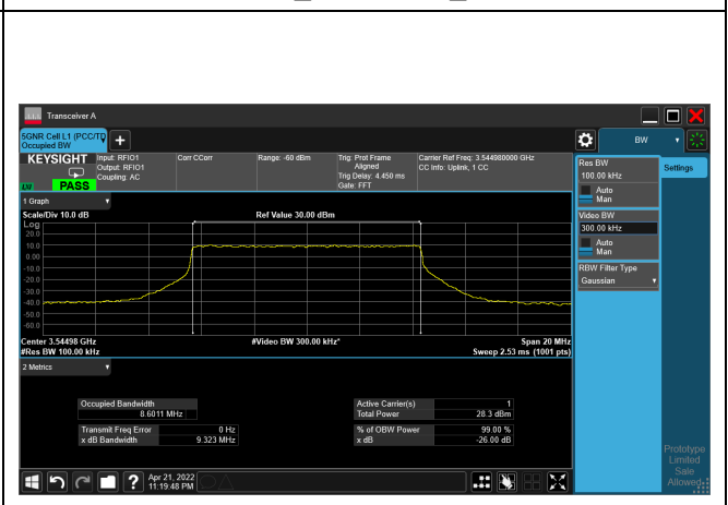
QPSK_CH636332_10M
