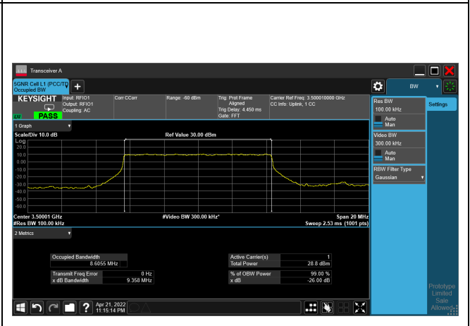
pi/2-BPSK_CH633334_10M
