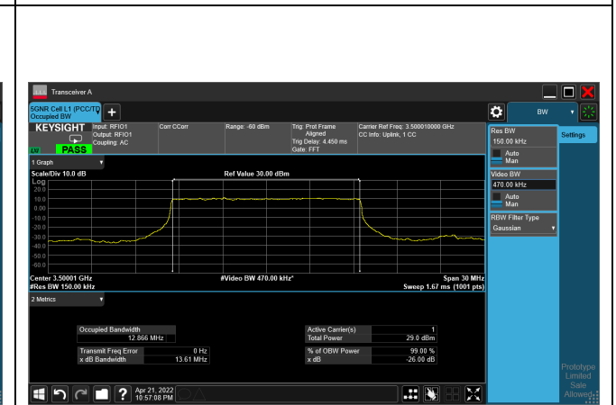
pi/2-BPSK_CH 633334_15M
