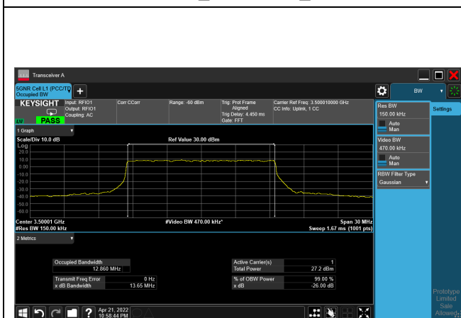
64QAM_CH633334_15M
