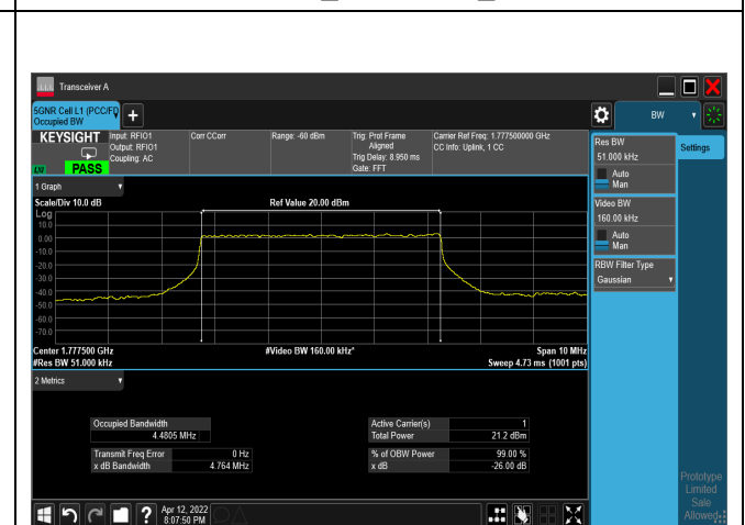
64QAM_CH355500_5M
