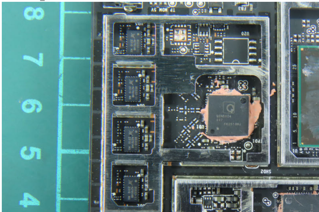
(28) EUT Photo_WIFI
