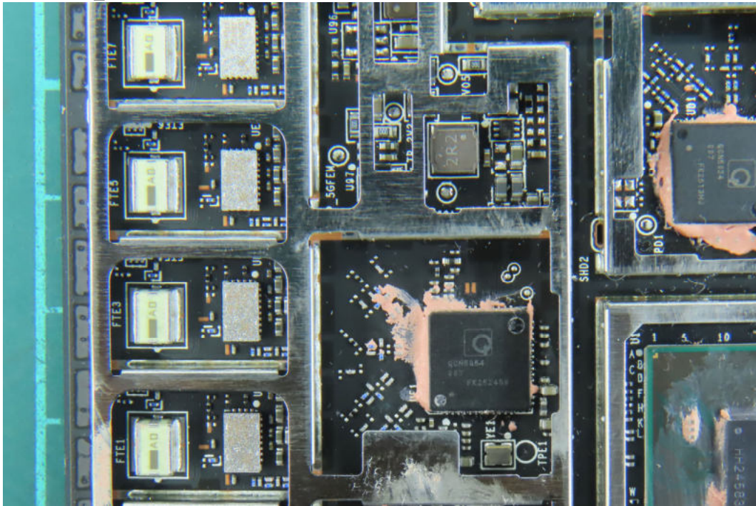
(31) EUT Photo_WIFI
