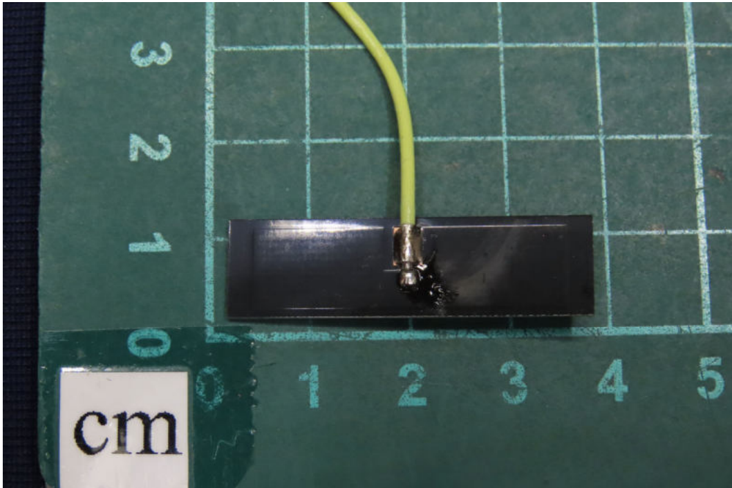
(47) EUT Photo (LV65C-LTE/FR1-S7)
