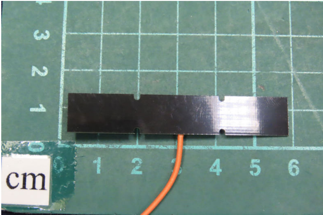
(49) EUT Photo (LV65C-LTE/FR1-S5)
