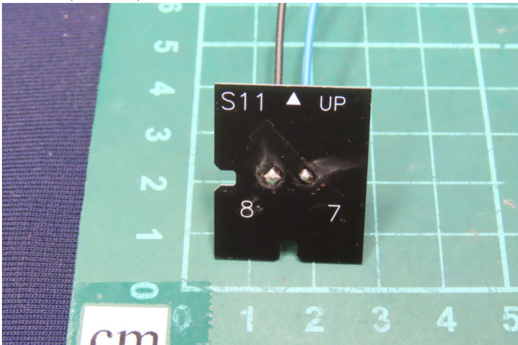
(58) EUT Photo (6E antenna)
