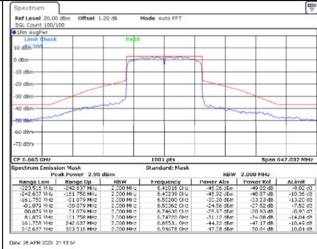
802.11ax160 / 6665MHz / Chain B - CDD
