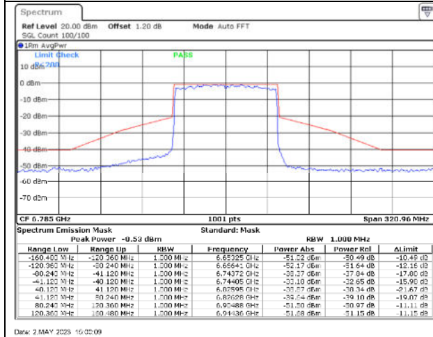
802.11ax80 / 6785MHz / Chain C - CDD
