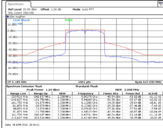
802.11ax160 / 6185MHz / Chain A - CDD
