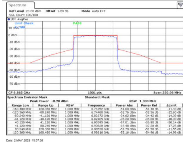
802.11ax80 / 6865MHz / Chain A - CDD
