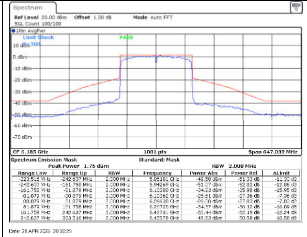
802.11ax160 / 6185MHz / Chain B - CDD
