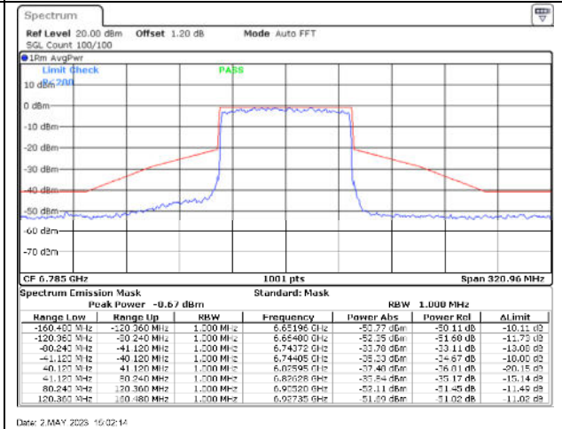
802.11ax80 / 6785MHz / Chain D - CDD
