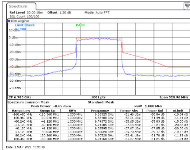
802.11ax80 / 6785MHz / Chain A - CDD
