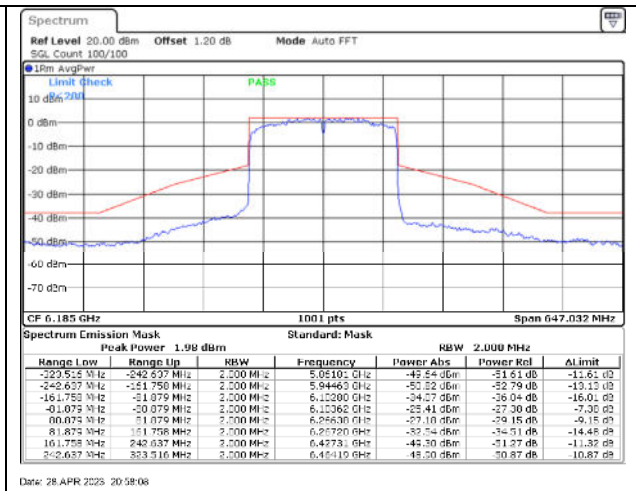
802.11ax160 / 6185MHz / Chain D - CDD
