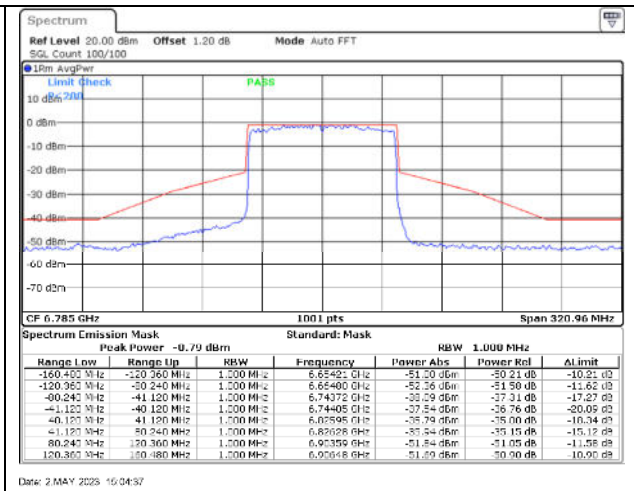
802.11ax80 / 6785MHz / Chain B - CDD
