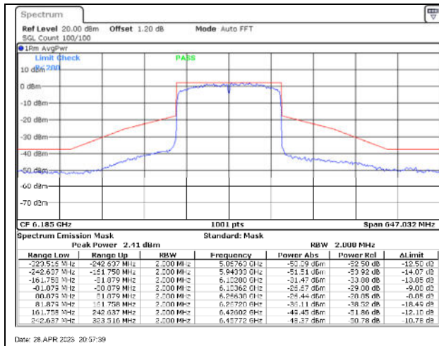
802.11ax160 / 6185MHz / Chain C - CDD
