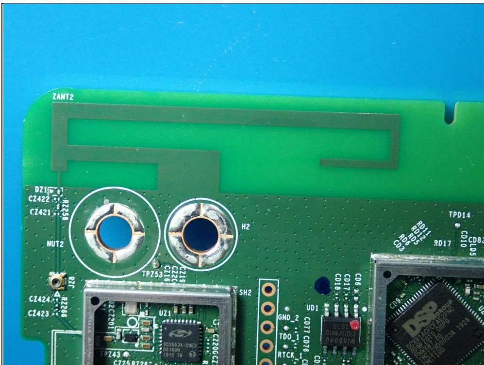
Antenna – Zwave
