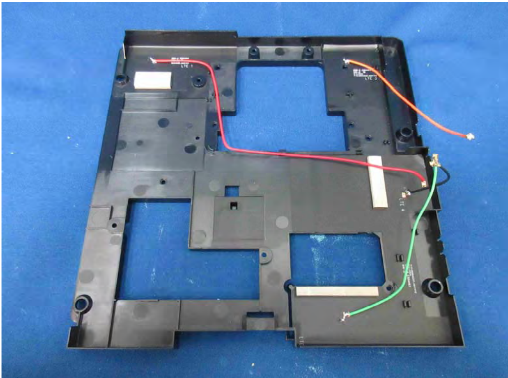
(62) EUT Photo
