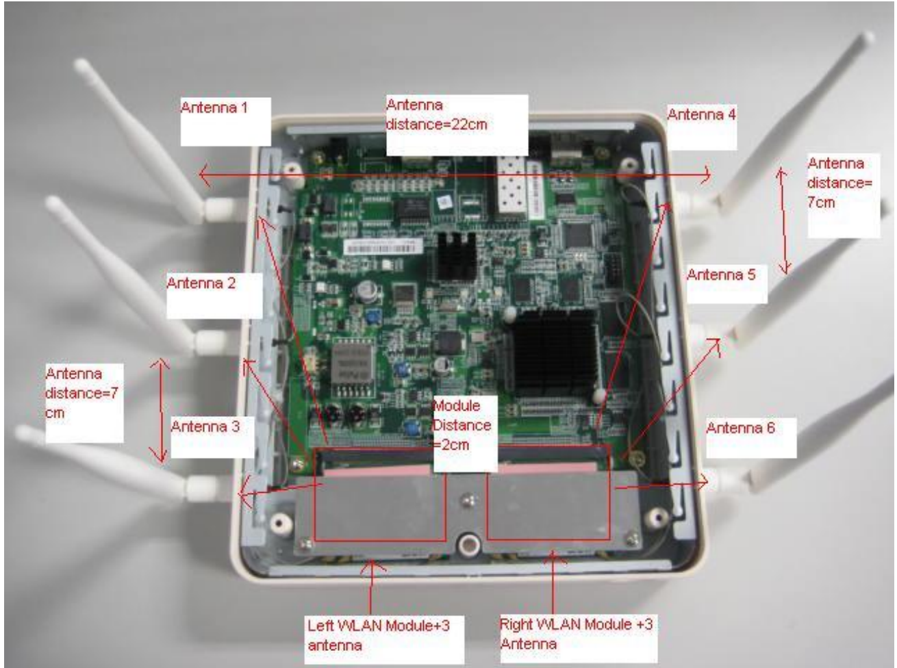
RG-AP220-E
