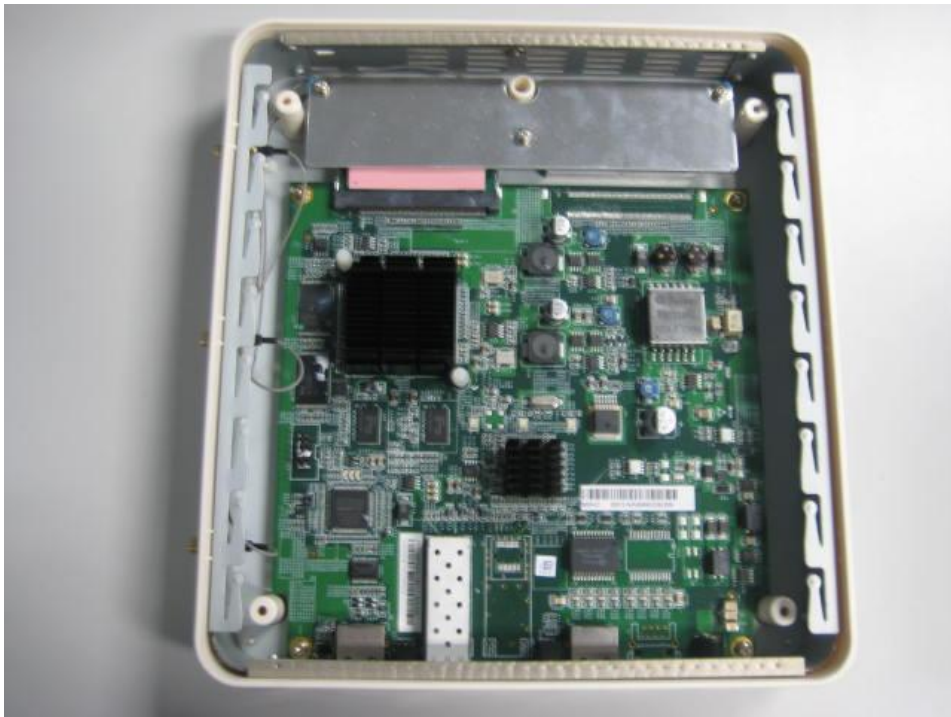
RG-AP220-SE
