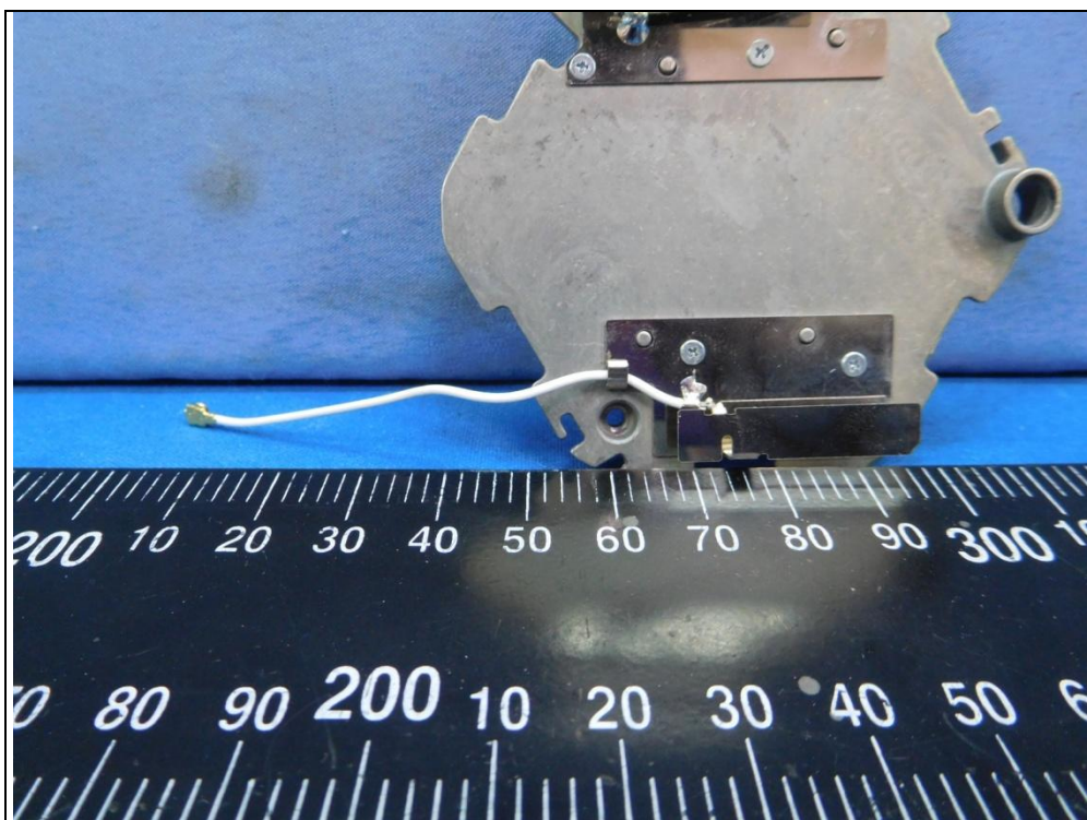
WLAN Ant. 1
