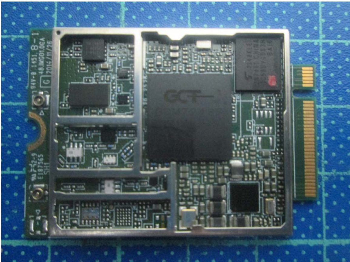
LTE Module
