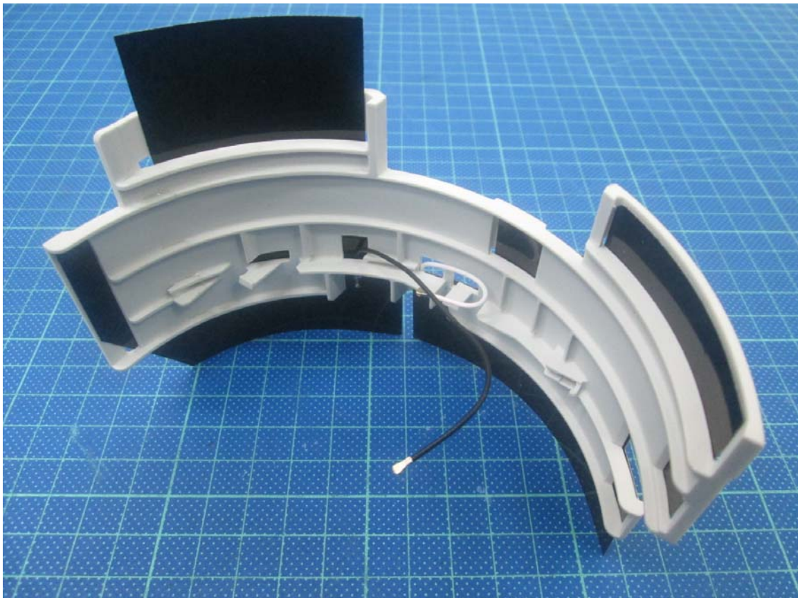
LTE antenna
