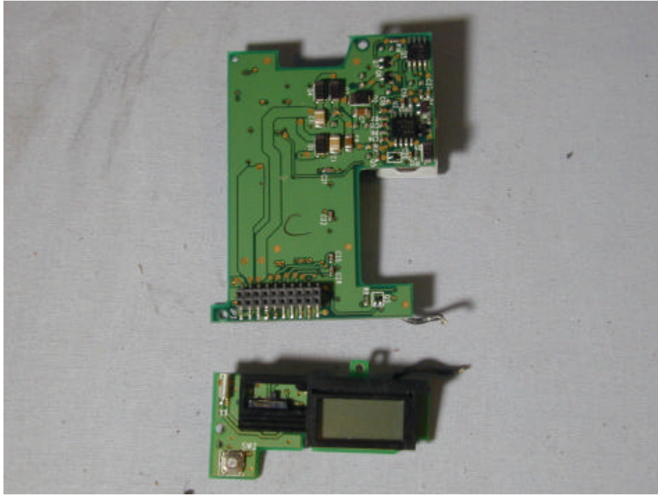
(14) EUT Photo
