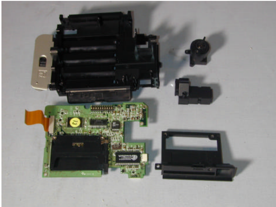
(24) EUT Photo
