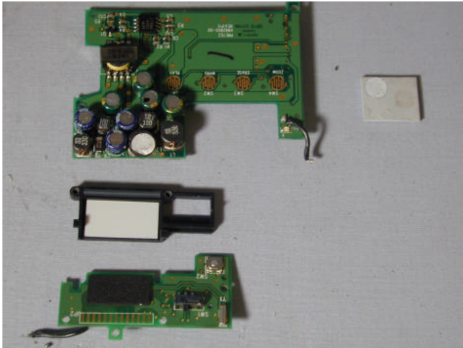
(16) EUT Photo
