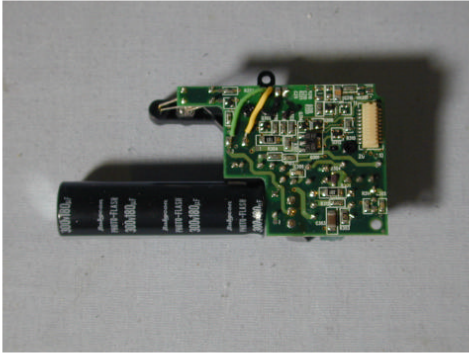
(20) EUT Photo
