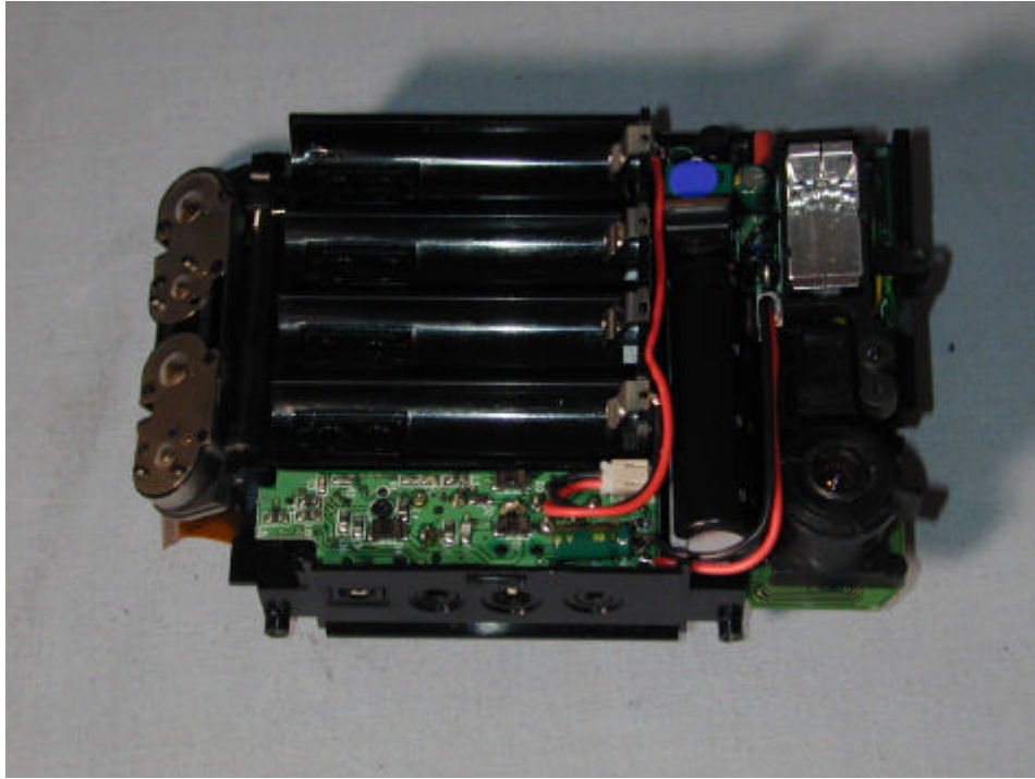
(18) EUT Photo
