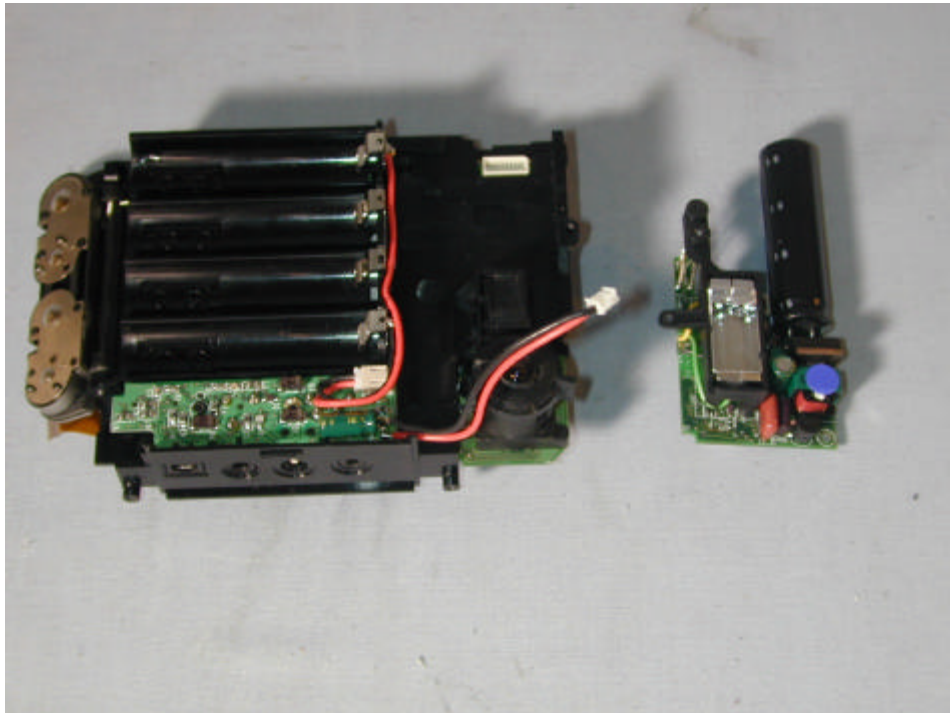
(18) EUT Photo
