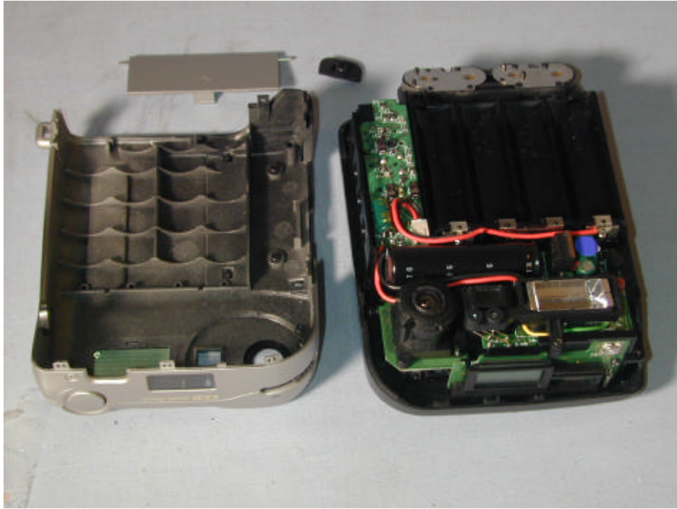
(8) EUT Photo
