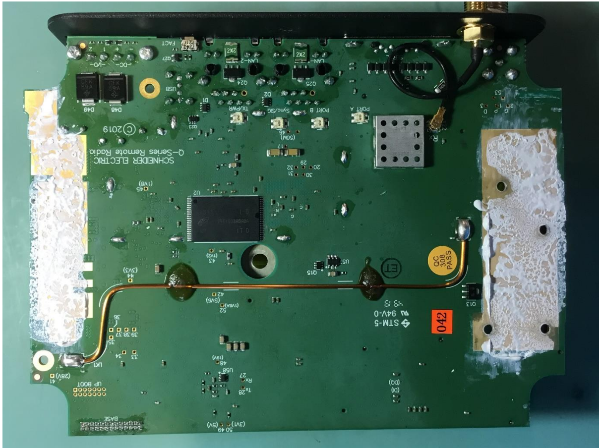
Radio PCB Bottom Layer
