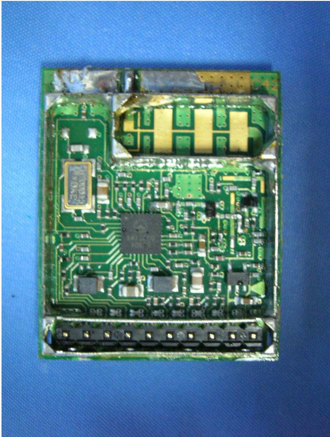
(8) EUT Photo
