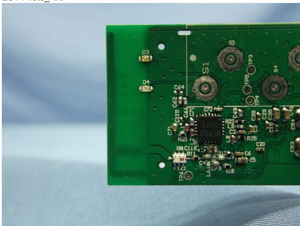
(19) EUT Photo_Ant
