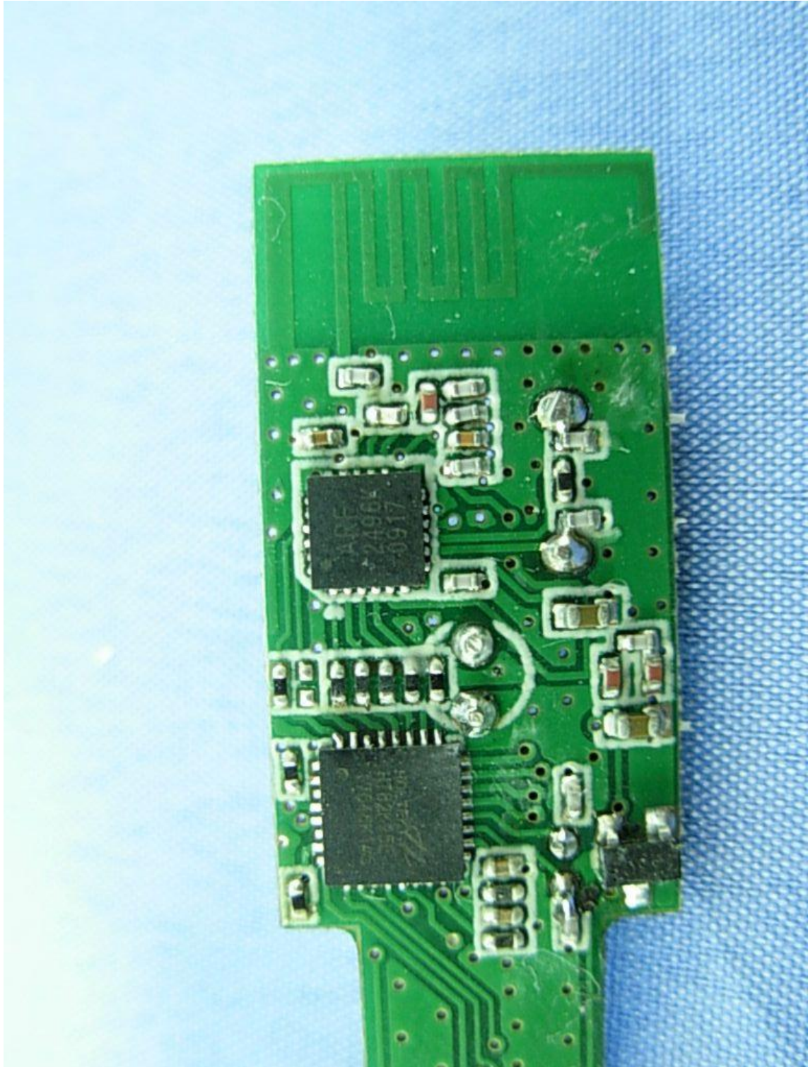
(10) EUT Photo
