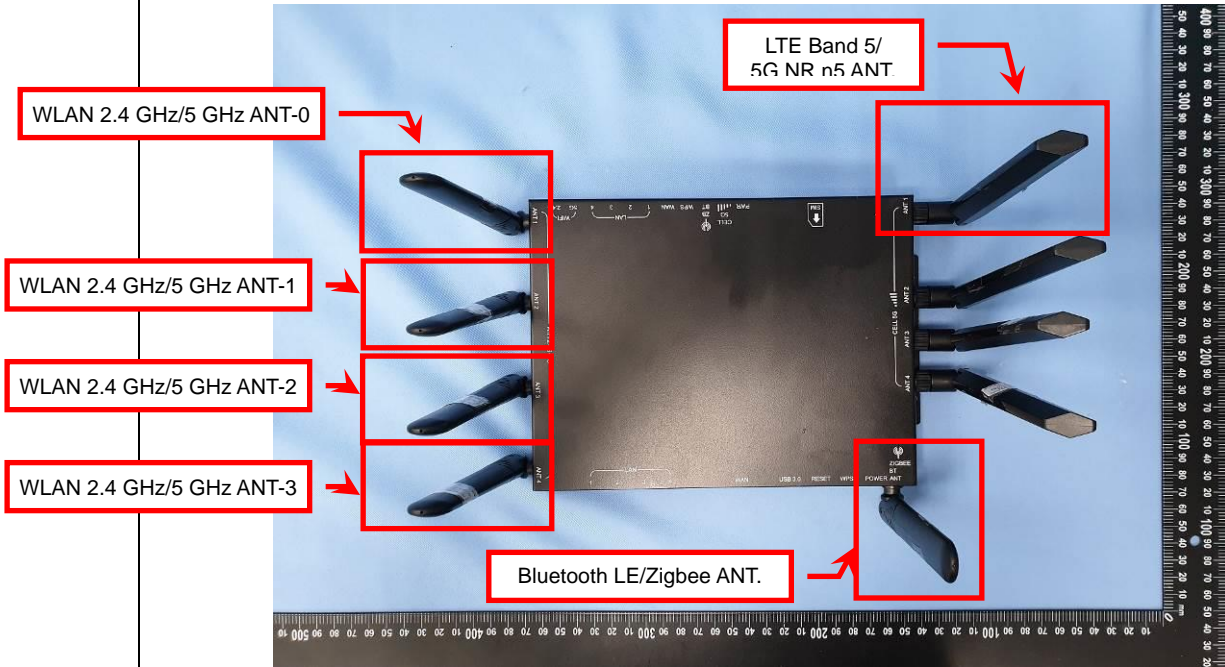
EUT Photo (2)
