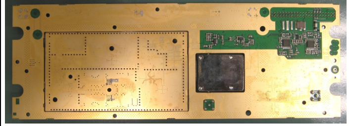
850MHz Amplifier Bottom
