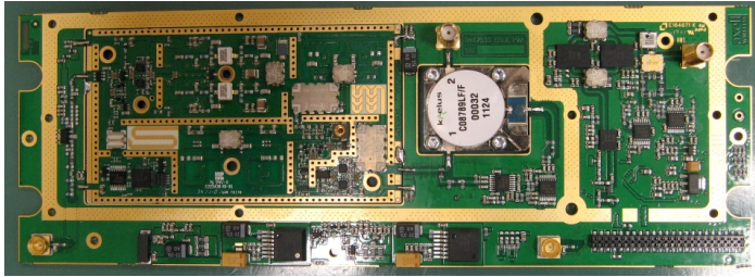
850MHz Amplifier Top
