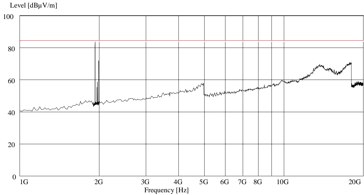
— MES cz_em_sc10 RE E-field ClassB, d=3m
