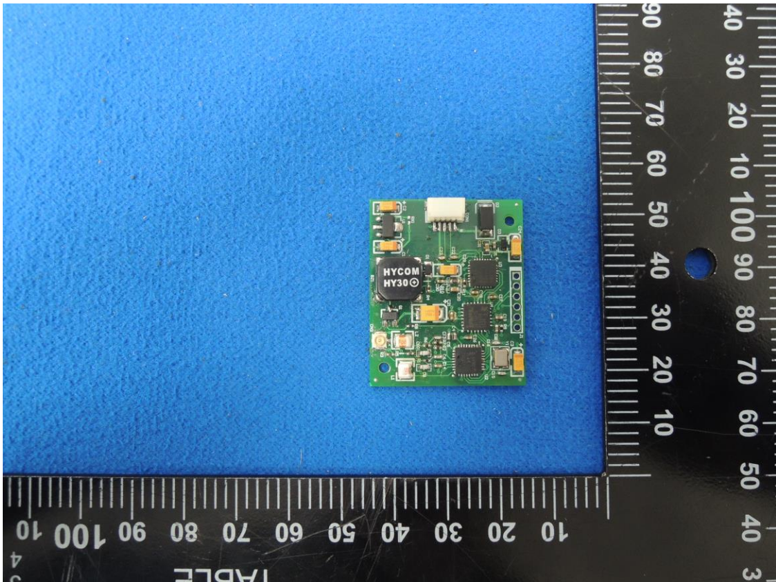
RFID Module
