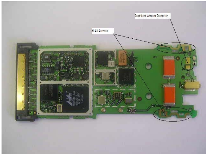
Antenna
