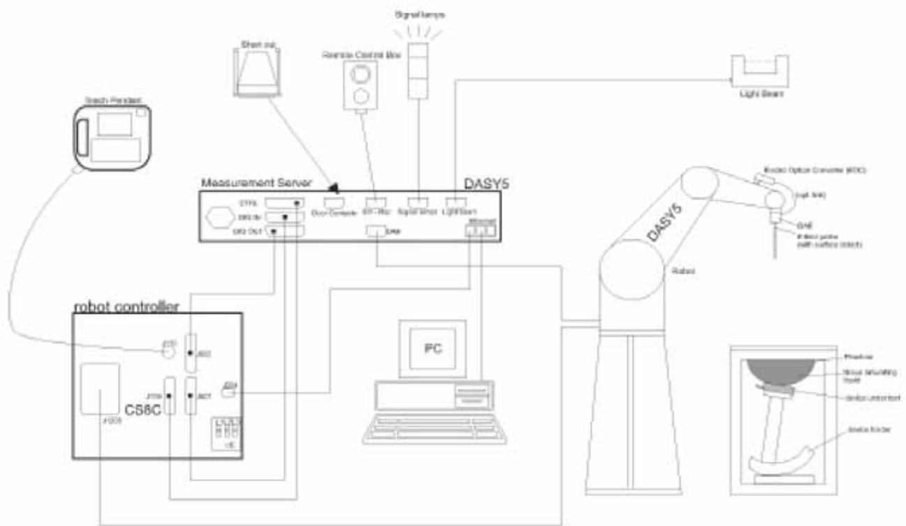
Fig. 5.1 DASY5 System
