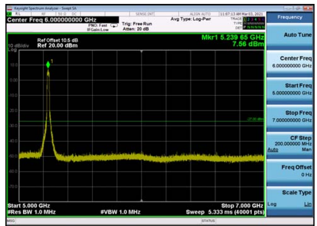
U-NII-1 ,Plot 3,5000MHz~7000MHz-802.1 1ac(40MHz),5230MHz
