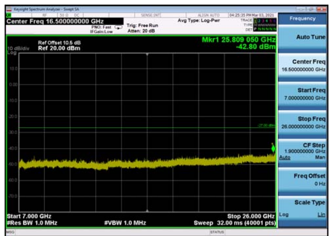
U-NII-3 ,Plot 4,7000MHz~26000MHz-802. 11a(20MHz),5825MHz
