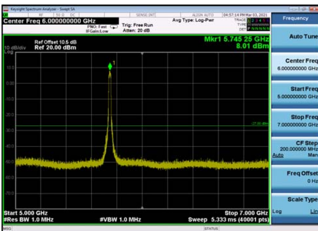
U-NII-3 ,Plot 3,5000MHz~7000MHz-802.1 n(20MHz),5745MHz
