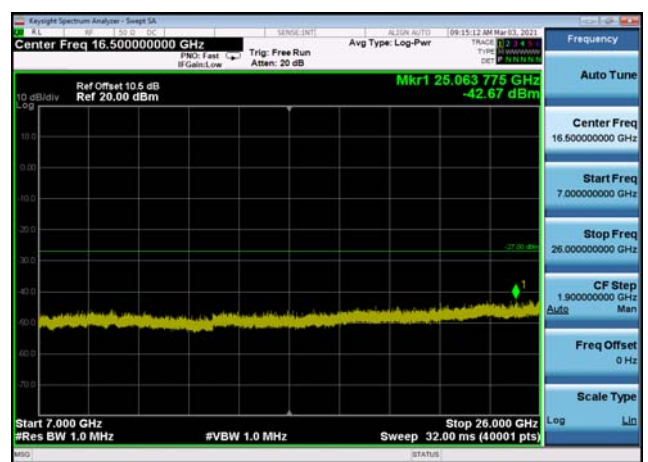
U-NII-1 ,Plot 4,7000MHz~26000MHz-802. 11a(20MHz),5180MHz
