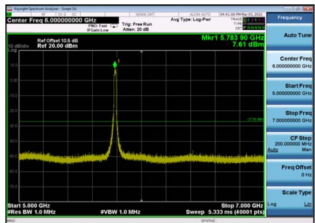
U-NII-3 ,Plot 3,5000MHz~7000MHz-802.1 n(20MHz),5785MHz
