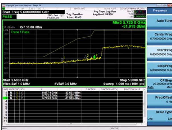
U-NII-3 ,Plot 1,Band Edge-802.11ac(80 MHz),5775MHz Left Side
