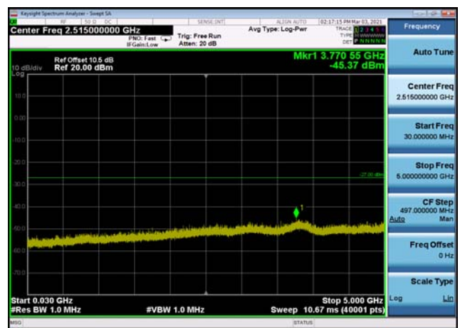
U-NII-1 ,Plot 2,30MHz~5000MHz-802.11a c(40MHz),5190MHz
