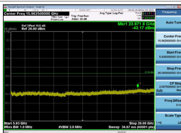
U-NII-3 ,Plot 3,5925MHz~26000MHz-802. 11ac(40MHz),5755MHz,Ant1
