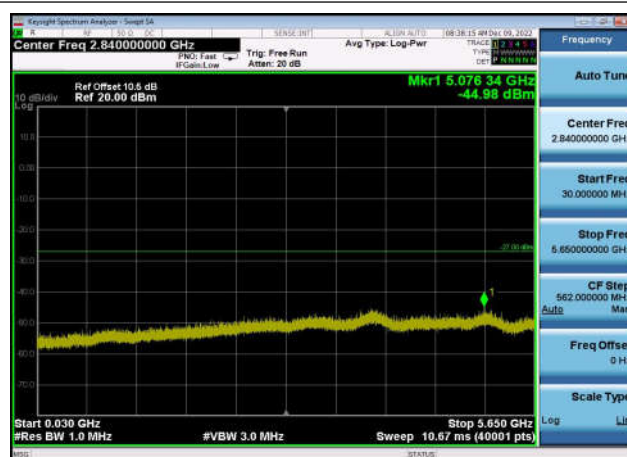
U-NII-3 ,Plot 2,30MHz~5650MHz-802.11a c(20MHz),5745MHz,Ant1
