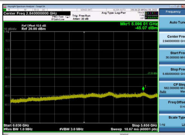
U-NII-3 ,Plot 2,30MHz~5650MHz-802.11a c(20MHz),5825MHz,Ant1
