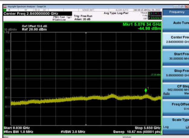
U-NII-3 ,Plot 2,30MHz~5650MHz-802.11a c(20MHz),5745MHz,Ant1
