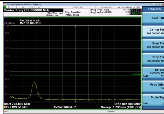
FDD13_10MHz_782_QPSK_OneRB_high_ExtraBands_Range_793~805
