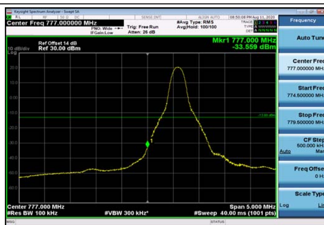
LowRange_FDD13_10MHz_782_OneRB_low_QPSK
