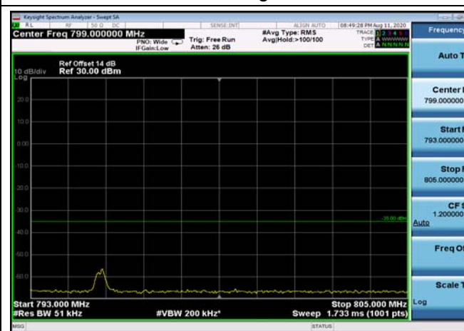
FDD13_10MHz_782_QPSK_OneRB_high_ExtraBands_Range_793-805
