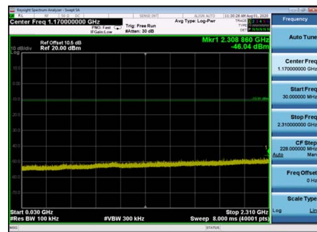
,Plot 3,30MHz~2310MHz-802.11b,2462MHz
