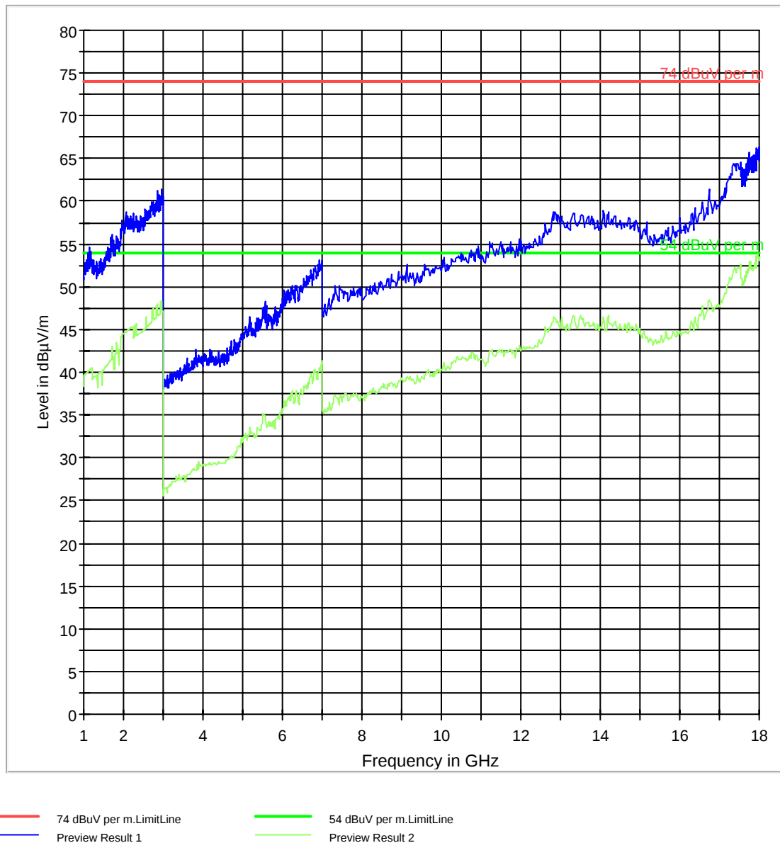
FCC 15 1-18GHz
