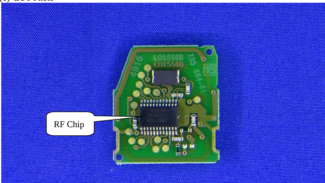
(6) EUT Photo
