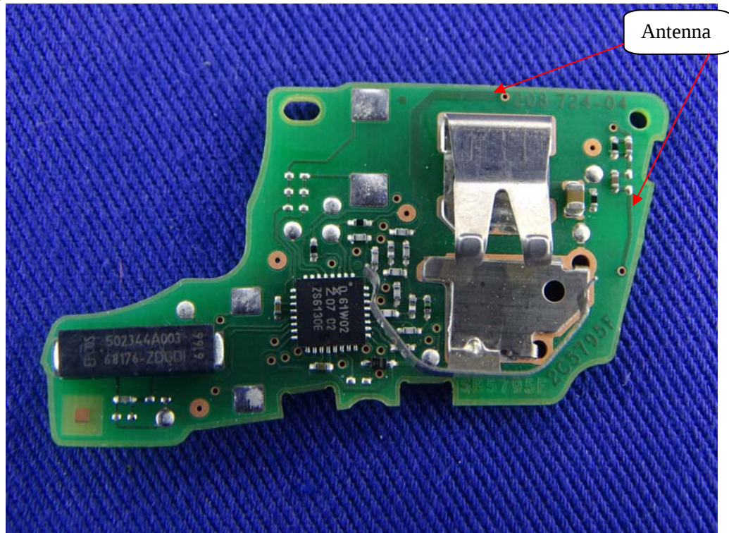
(16) EUT Photo
