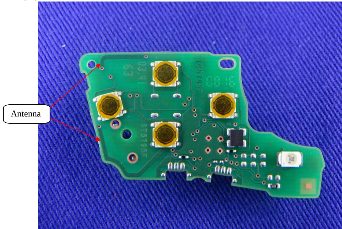
(17) EUT Photo
