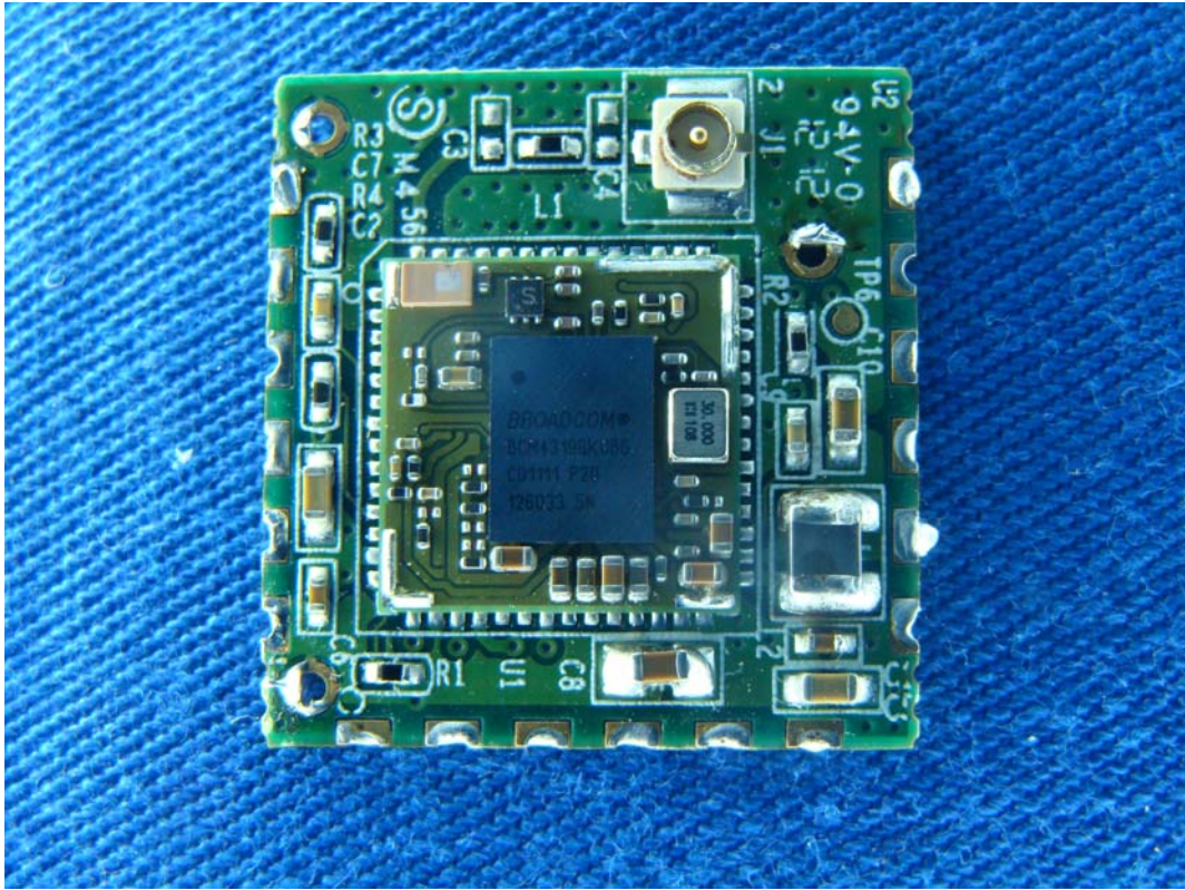
(17) EUT Photo (WLAN Module)
