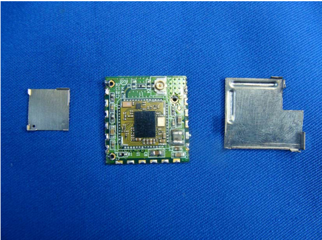
(16) EUT Photo (WLAN Module)
