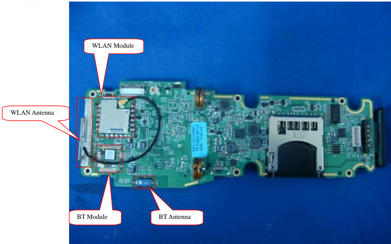
(9) EUT Photo
