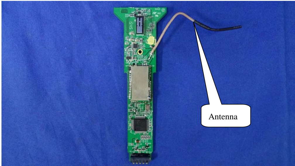
(4) EUT Photo
