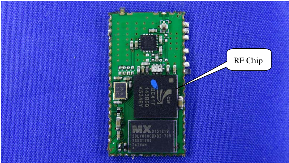
(8) EUT Photo
