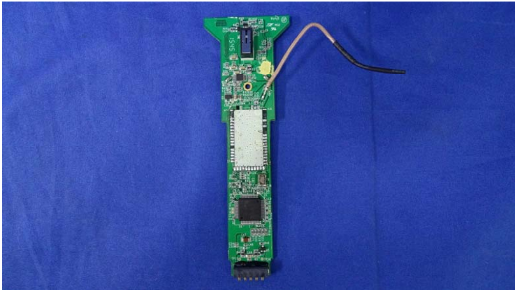
(10) EUT Photo
