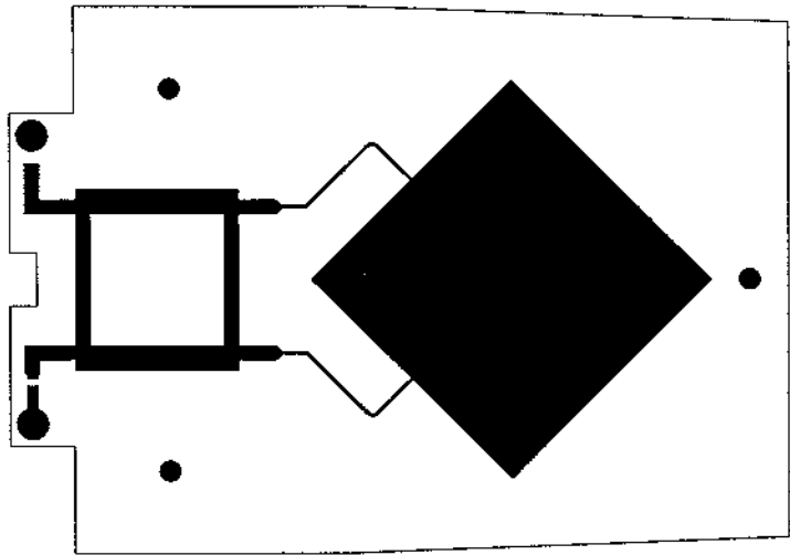
LAYER 1 (PRIMARY SIDE)
