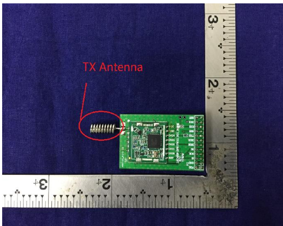
(2) EUT Photo
